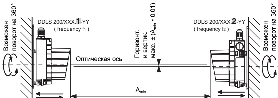
Рис. 4.1: Монтаж устройств
