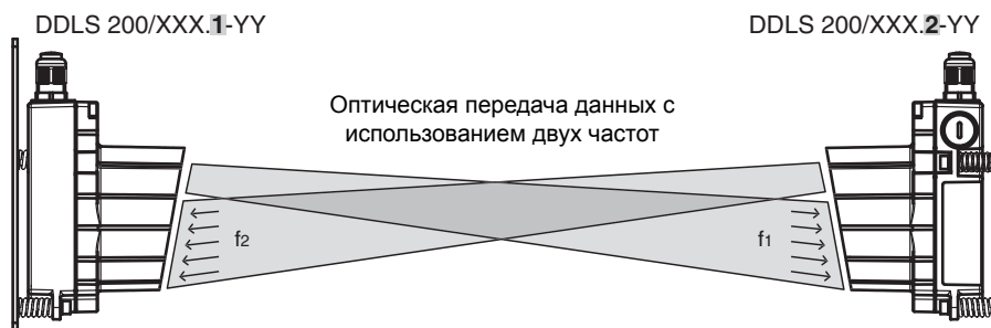
Рис. 1.1: Принцип действия
