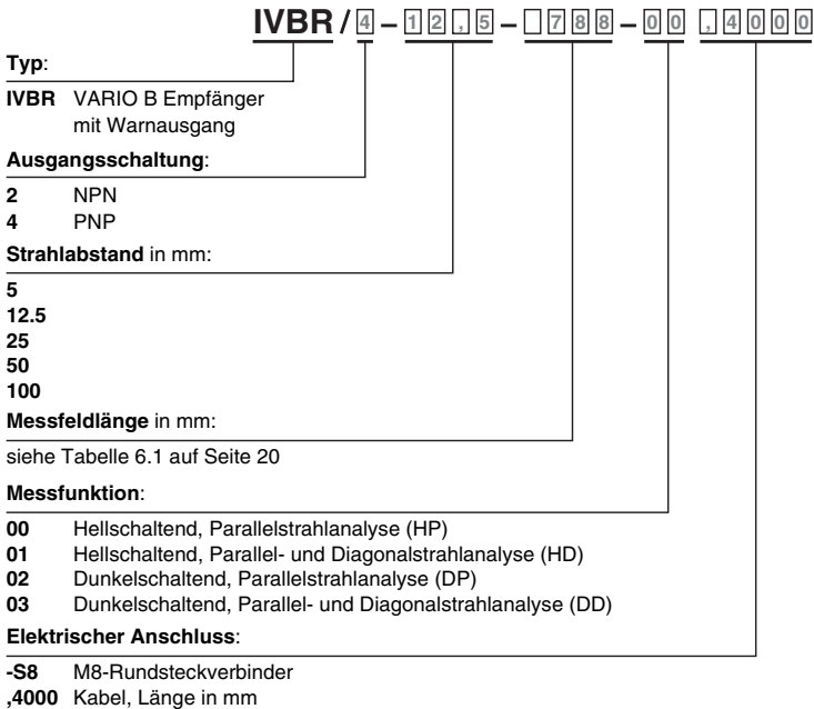
Bild 6.2: Typenschlüssel VARIO B Empfänger
