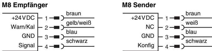
Bild 4.2: Anschlussbelegung M8-Steckverbinder des VARIO B-Lichtvorhangs
