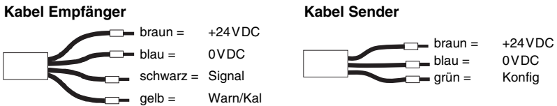
Bild 4.3: Anschlussbelegung Kabel des VARIO B-Lichtvorhangs
