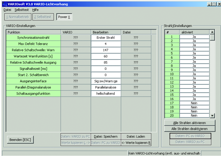
Bild 3.2: Parametrierfenster von VARIOSoft 3.1:
