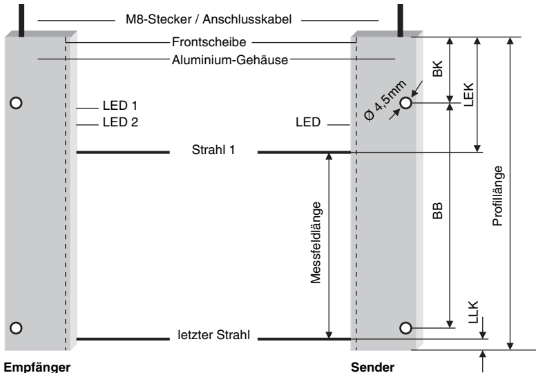
Bild 4.1: Montage des VARIO B-Lichtvorhangs
