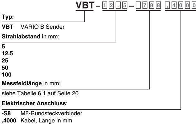
Bild 6.1: Typenschlüssel VARIO B Sender
