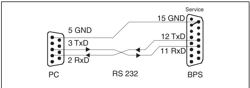
圖 7.1: 連接維修操作介面到 PC 或終端機
