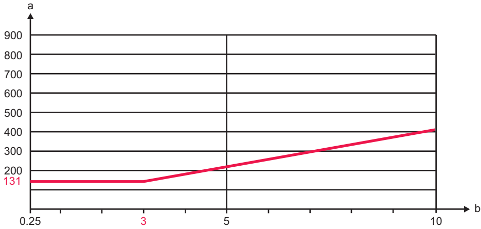
Resim 4.2: Yansıyan yüzeylere doğru olan minimum mesafe
