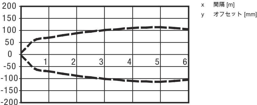
典型的な応答挙動 ( TK 100x100 )
