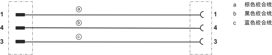
接线图
