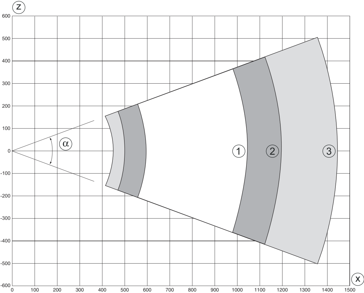
Krzywa pola odczytu Low Density
