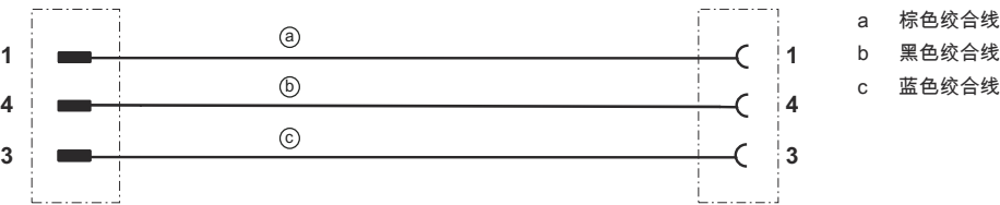
接线图
