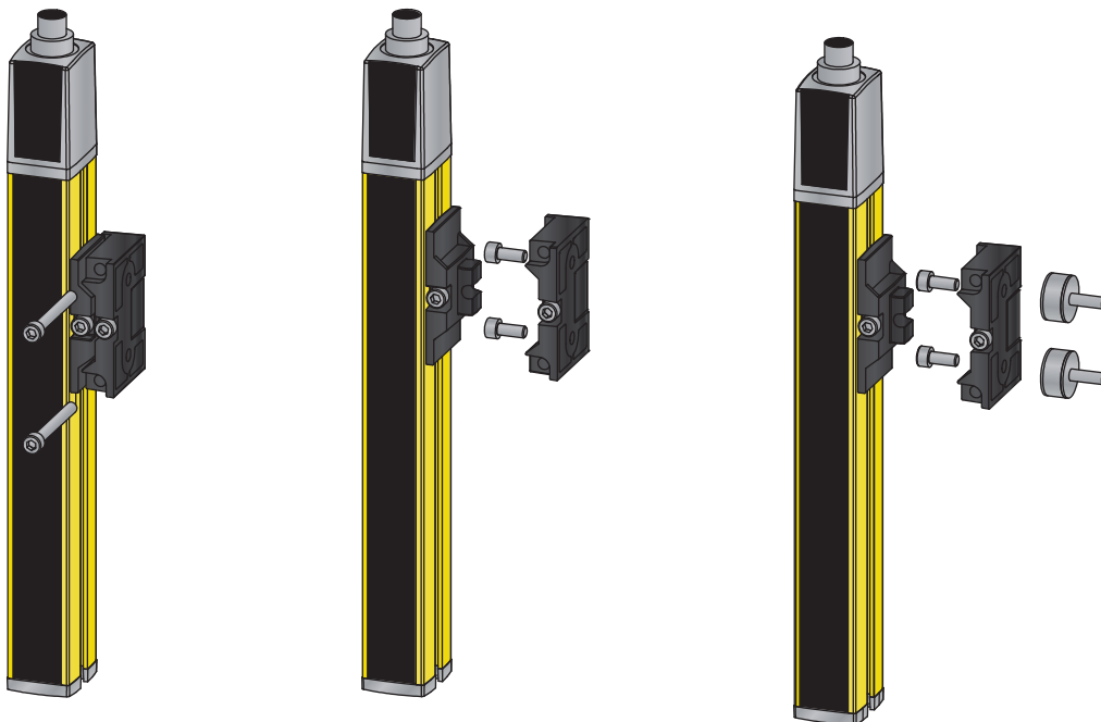
Figura 6.9: Montaje a través de soporte orientable BT-2SB10
