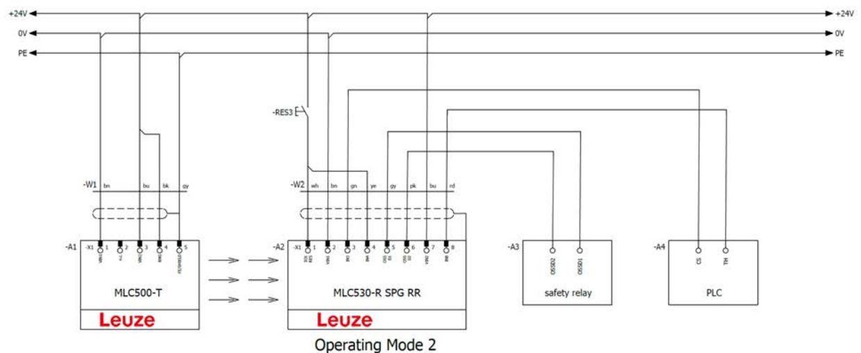
Bild 8.34: Betriebsart 2: Schaltungsbeispiel mit Smart Process Gating (SPG)
