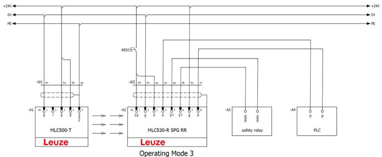
Bild 8.35: Betriebsart 3: Schaltungsbeispiel mit Smart Process Gating (SPG)
