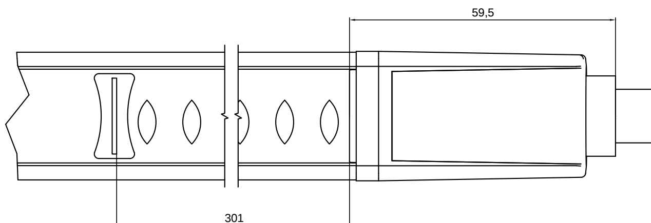
Bild 15.2: Position Auflösungsgrenzen, an gekennzeichneteter Position findet der Auflösungswechsel statt.
