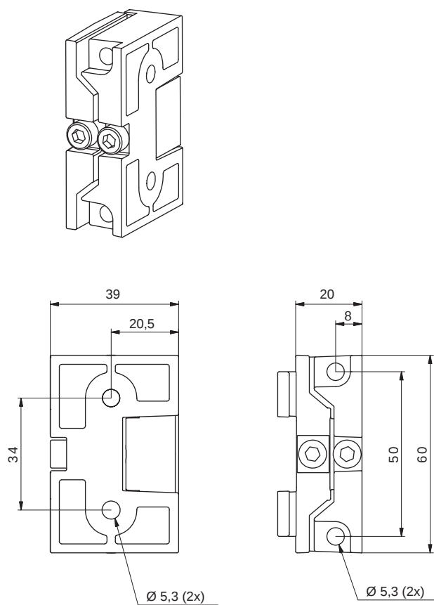
Bild 15.6: Schwenkhalterung BT-2SB10
