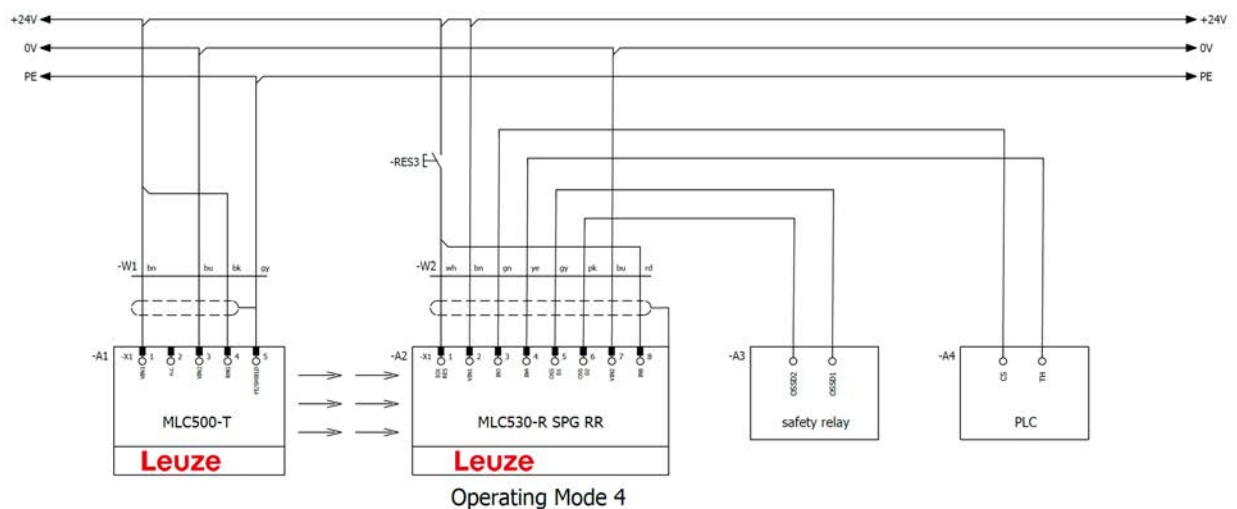
Bild 8.36: Betriebsart 4: Schaltungsbeispiel mit Smart Process Gating (SPG)
