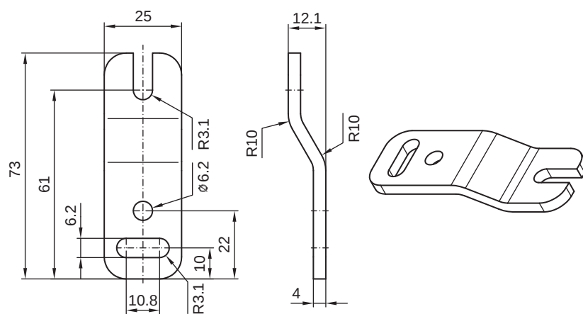
Bild 15.4: Parallelhalterung BT-Z
