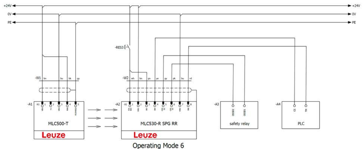
Bild 8.38: Betriebsart 6: Schaltungsbeispiel mit Smart Process Gating (SPG)
