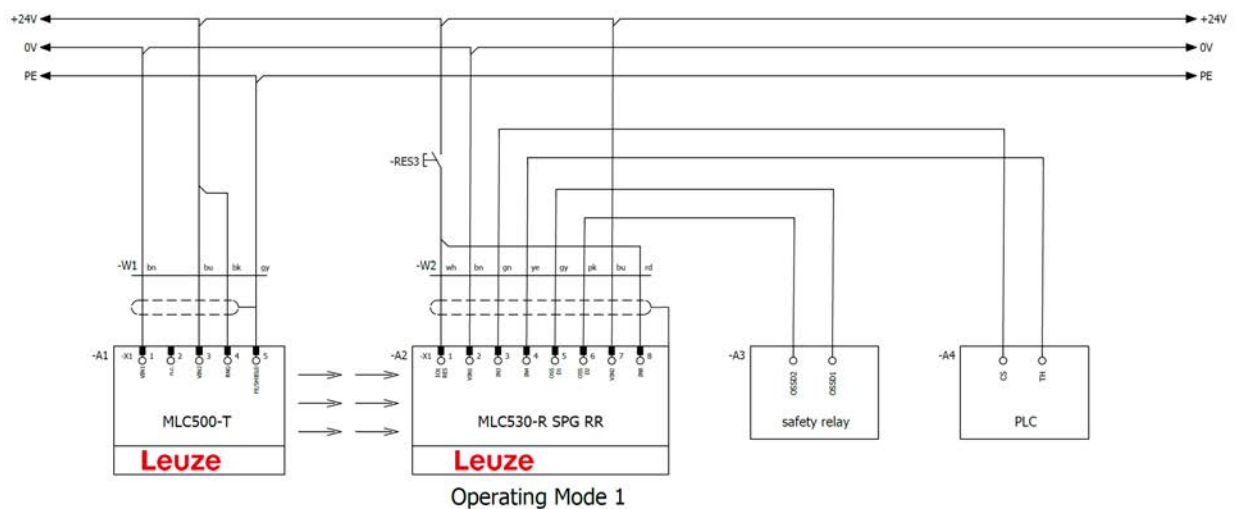
Bild 8.33: Betriebsart 1: Anschlussbeispiel mit Smart Process Gating (SPG)
