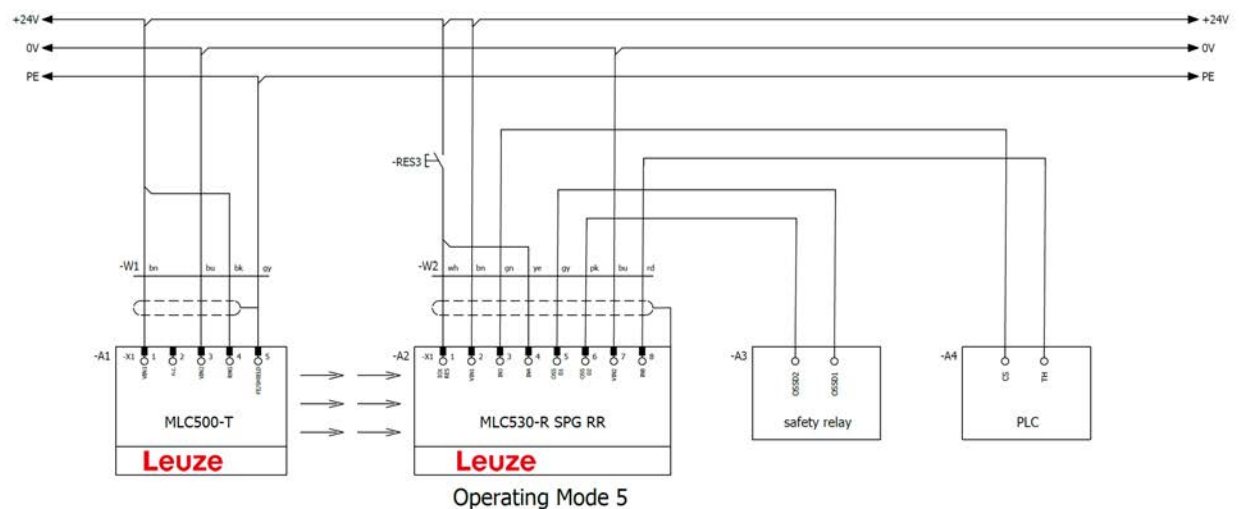
Bild 8.37: Betriebsart 5: Schaltungsbeispiel mit Smart Process Gating (SPG)
