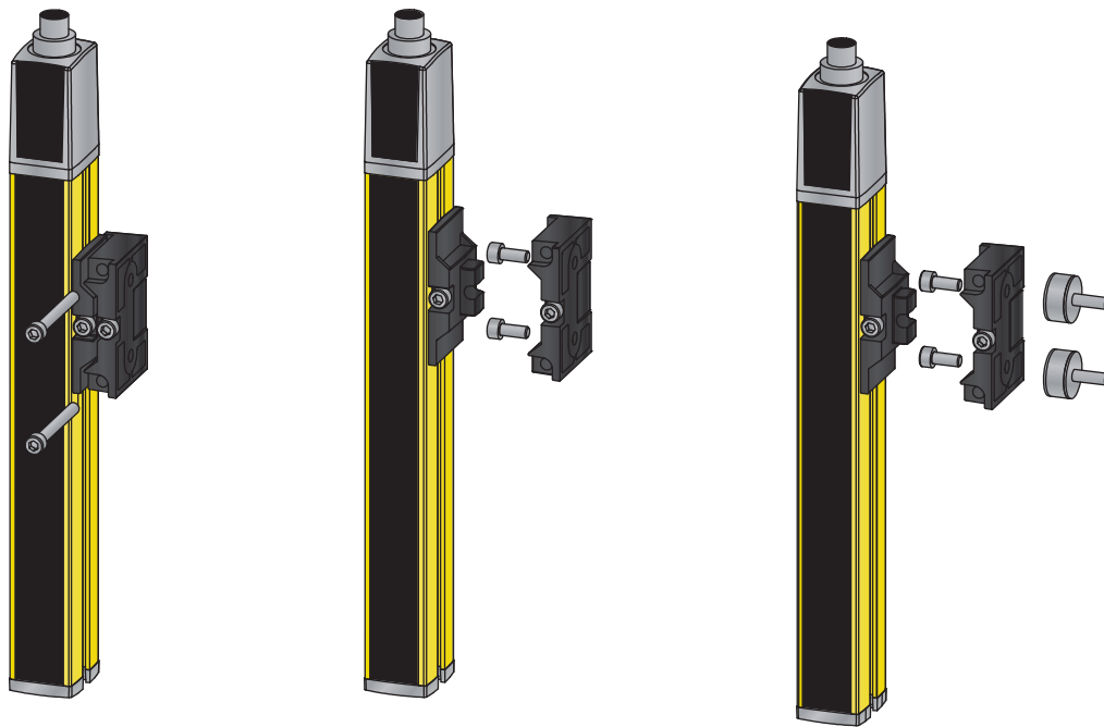
Bild 7.9: Montage über schwenkbare Halter BT-2SB10
