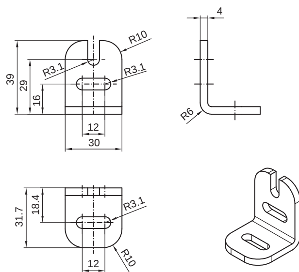
Bild 15.3: Winkelhalterung BT-L
