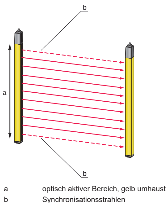
Bild 3.1: Sender-Empfänger-System
