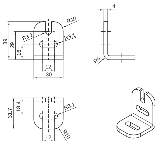
Bild 14.2: Winkelhalterung BT-L
