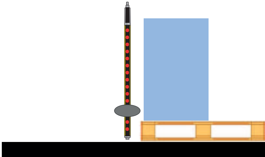
Figura 4.3: Interrupción del campo de protección con una resolución reducida y un objeto en el campo de protección. La resolución reducida está activa antes y después del gating.
