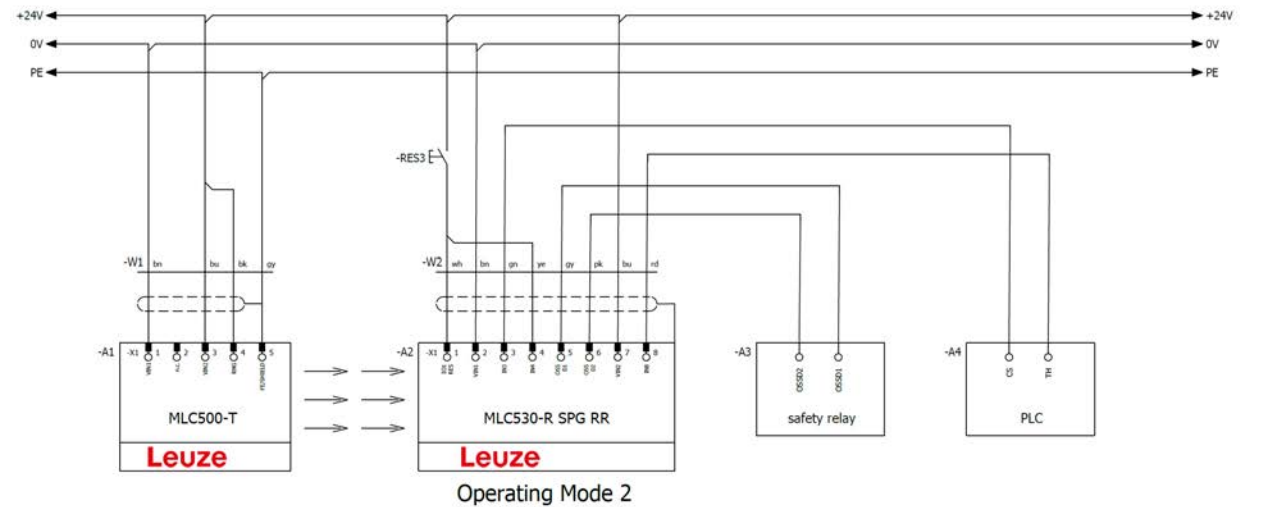
Figura 8.34: Modo de funcionamiento 2: ejemplo de circuito con Smart Process Gating (SPG)
