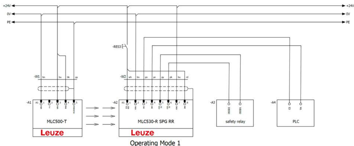
Figura 8.33: Modo de funcionamiento 1: ejemplo de conexión con Smart Process Gating (SPG)
