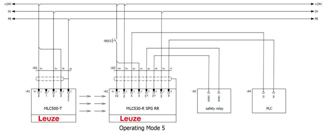
Figura 8.37: Modo de funcionamiento 5: ejemplo de circuito con Smart Process Gating (SPG)
