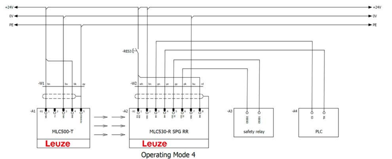
Figura 8.36: Modo de funcionamiento 4: ejemplo de circuito con Smart Process Gating (SPG)
