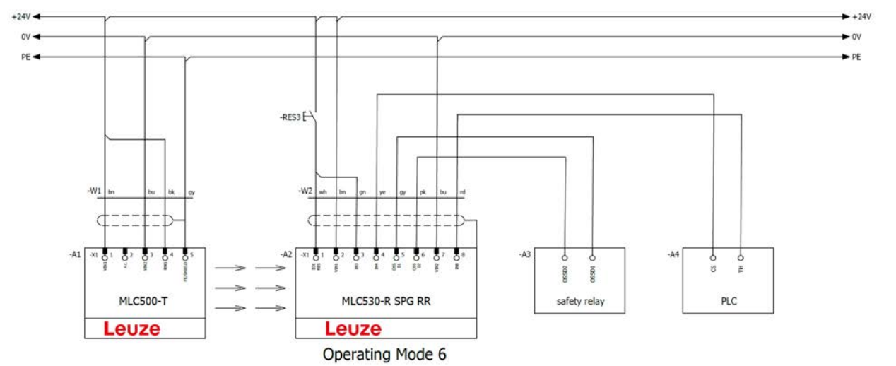
Figura 8.38: Modo de funcionamiento 6: ejemplo de circuito con Smart Process Gating (SPG)
