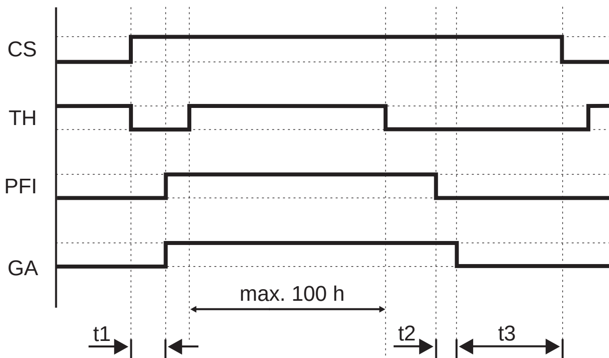
Figura 4.11: Prolongación del timeout de SPG
