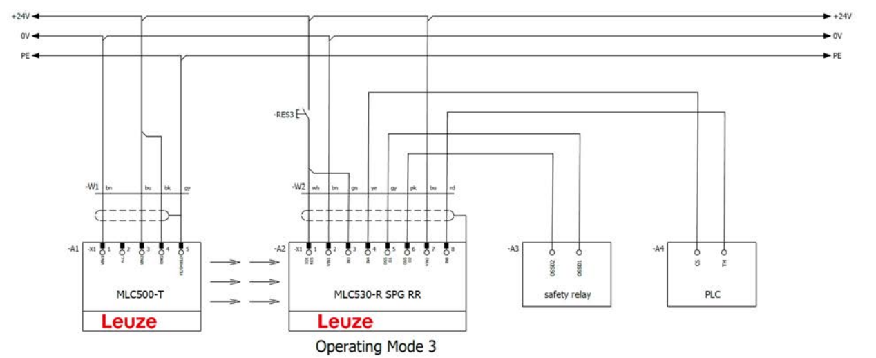
Figura 8.35: Modo de funcionamiento 3: ejemplo de circuito con Smart Process Gating (SPG)
