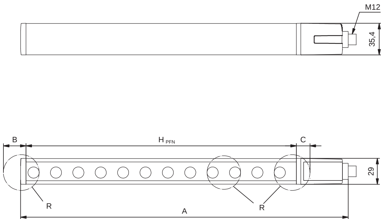
Figura 14.1: Medidas del emisor y receptor La altura del campo de protección efectiva H_{PFE} sale de las medidas del área óptica hasta los bordes exteriores de los círculos marcados con R.
