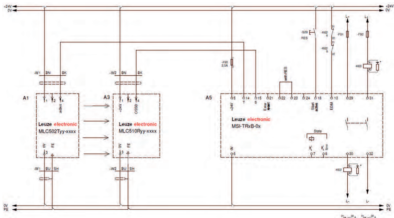
Bild 7.5: Schaltungsbeispiel mit externem Testgerät MSI-TRxB-0x mit EDM
