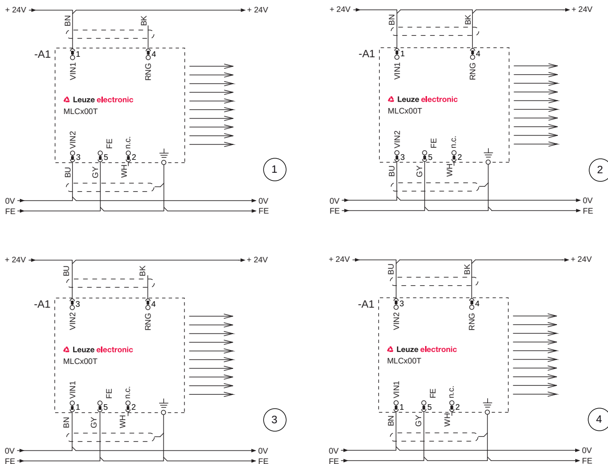
Bild 7.2: Anschlussbeispiele Sender
