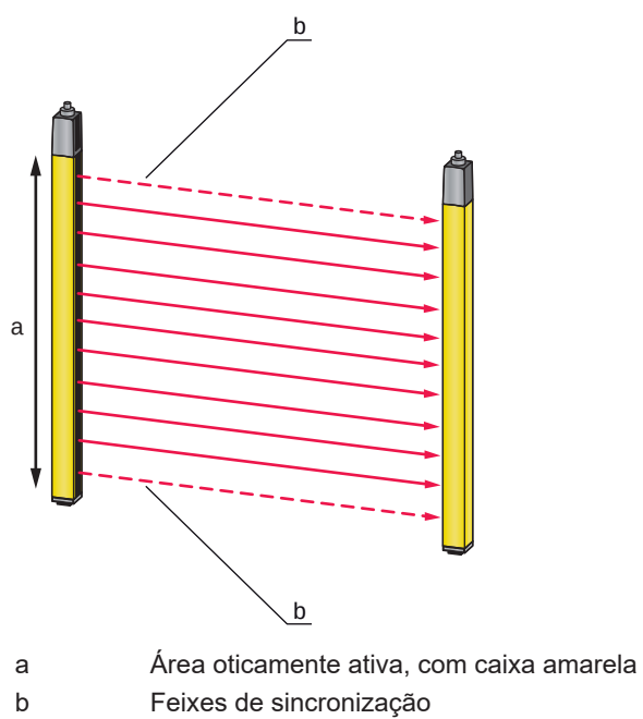
Fig. 3.1: Sistema transmissor/receptor
