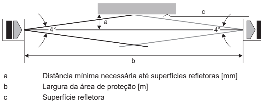
Fig. 6.2: Distância mínima até superfícies refletoras dependendo da largura da área de proteção
