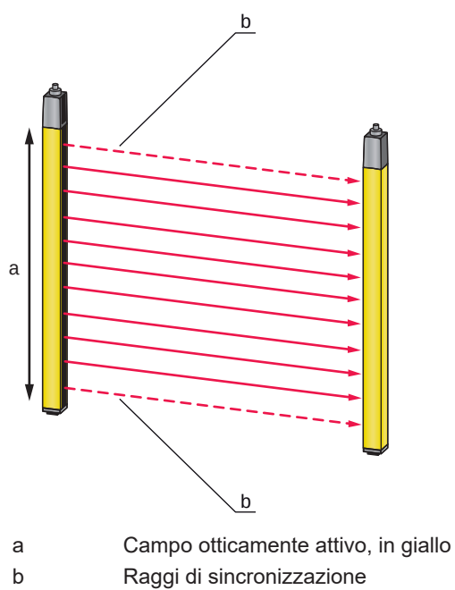
Figura 3.1: Sistema trasmettitore-ricevitore
