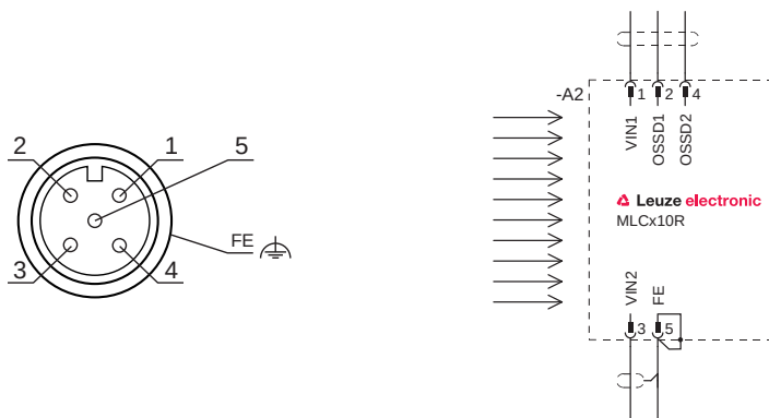
Figura 7.3: Assegnazione dei pin e schema di collegamento ricevitore
