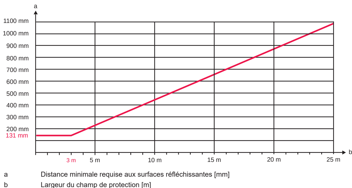
Fig. 6.3: Distance minimale aux surfaces réfléchissantes en fonction de la largeur du champ de protection
