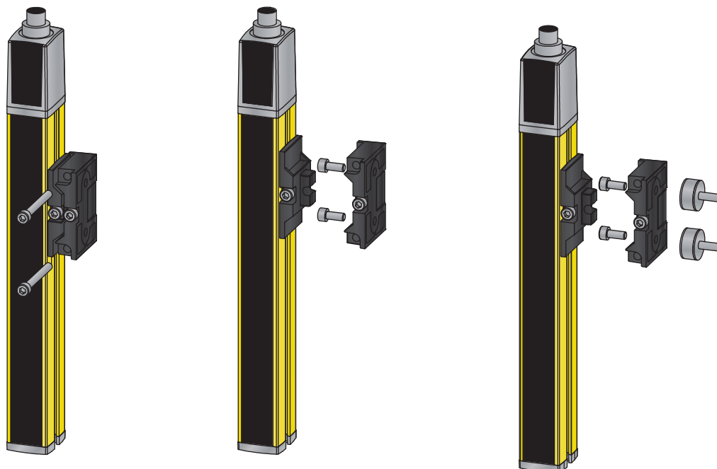
Fig. 6.9: Montage à l'aide de supports pivotants BT-2SB10
