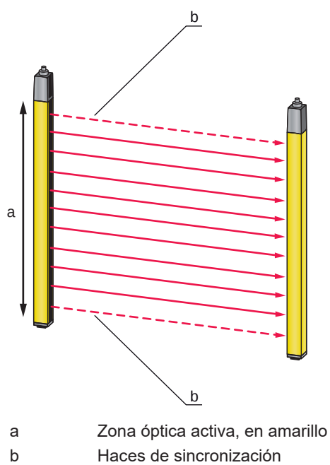
Figura 3.1: Sistema emisor-receptor
