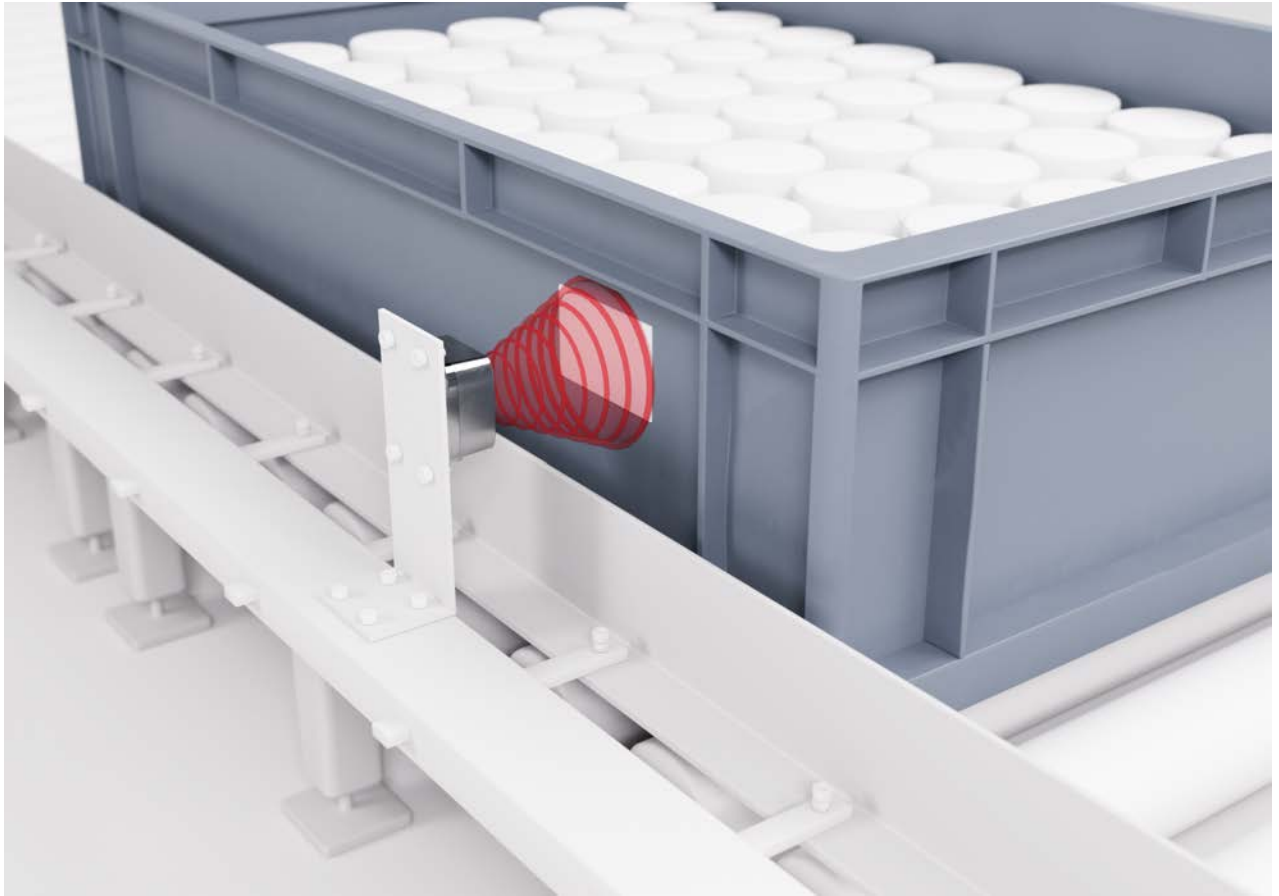
Resim 5.1: Konveyör hattı üzerindeki konteynerlerin tanımlanması
