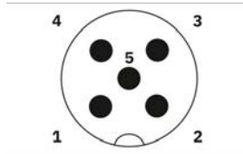
Figura 7.1: Conector M12 de 5 polos, con codificación A
