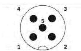
Figura 7.1: Connettore maschio M12 a 5 poli (codifica A)
