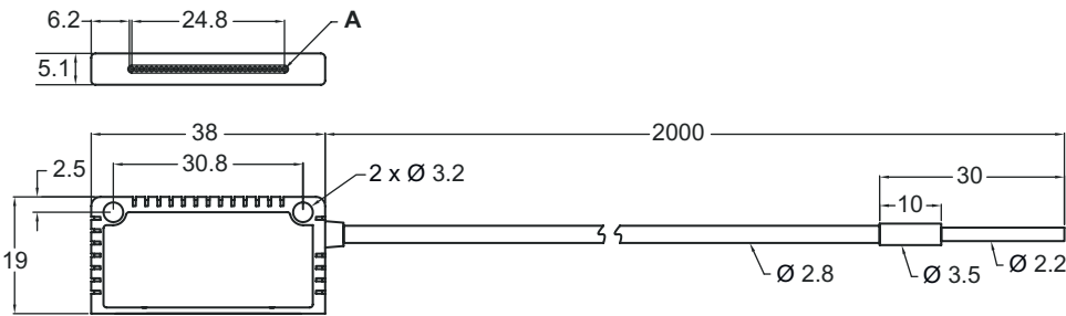
A Ø 0,265 mm núcleo de fibra de vidrio x 32 uds.
