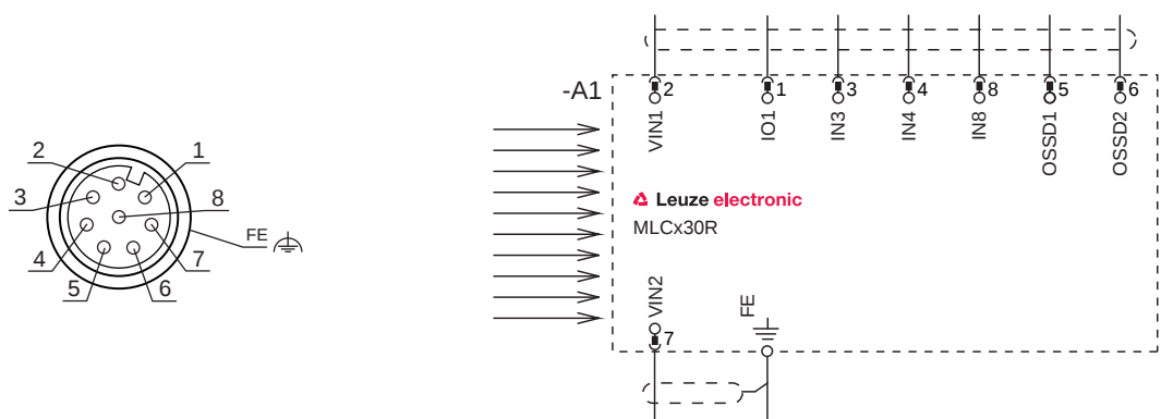
Bild 8.3: Steckerbelegung und Anschlussbild Empfänger
