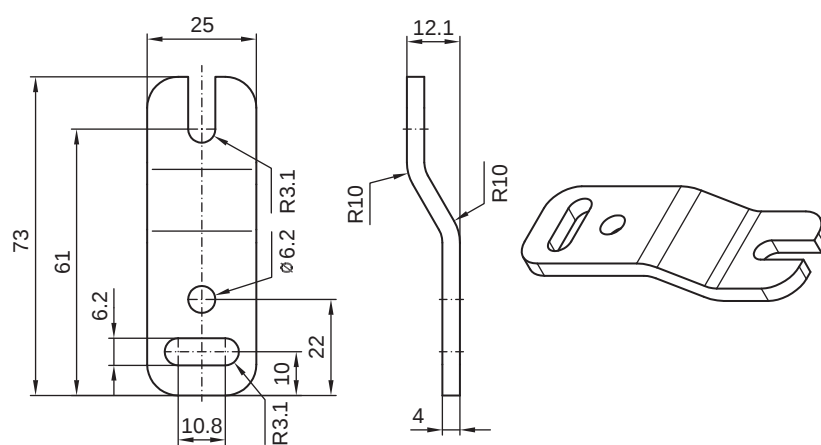
Bild 15.4: Parallelhalterung BT-Z
