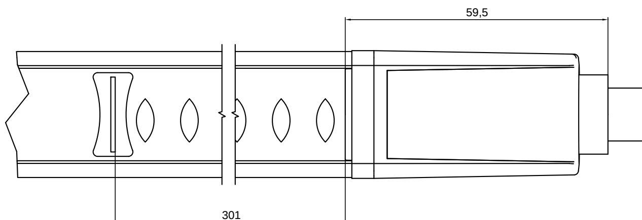
Bild 15.2: Position Auflösungsgrenzen, an gekennzeichneten Position findet der Auflösungswechsel statt.
