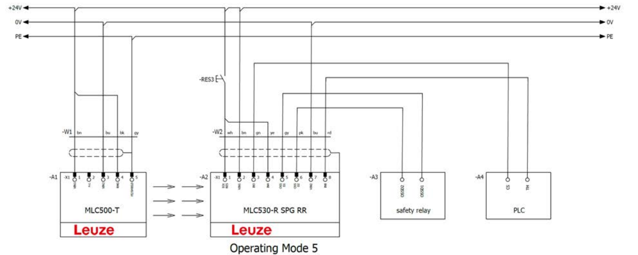
Figura 8.37: Modo operativo 5: esempio di collegamento con Smart Process Gating (SPG)
