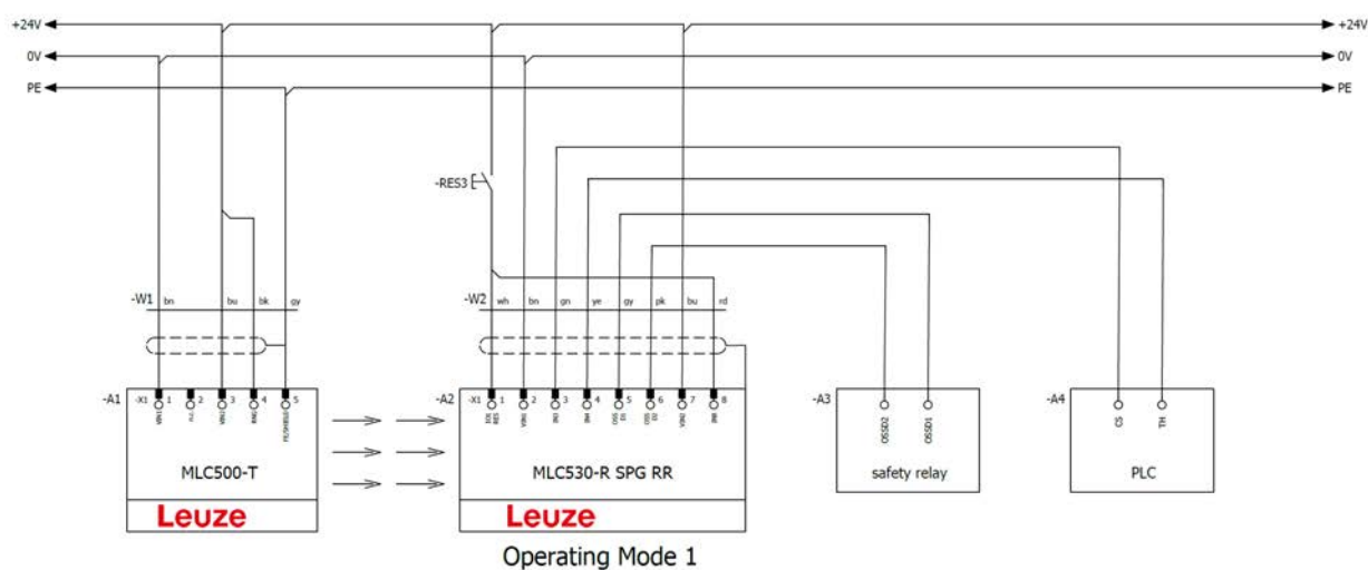
Figura 8.33: Modo operativo 1: esempio di collegamento con Smart Process Gating (SPG)
