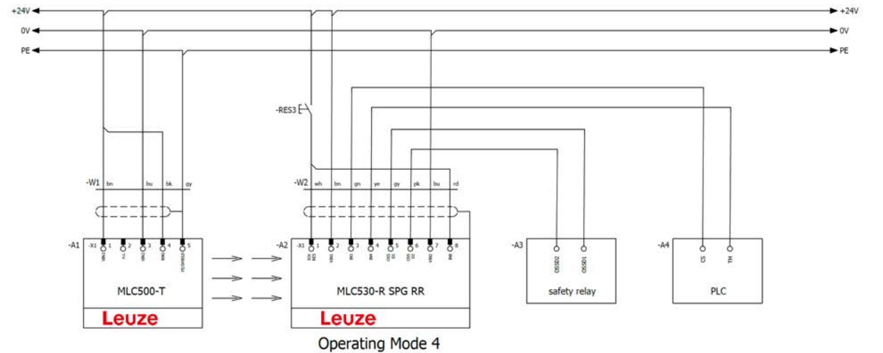
Figura 8.36: Modo operativo 4: esempio di collegamento con Smart Process Gating (SPG)
