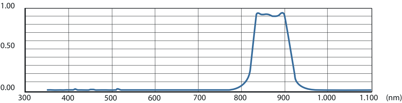
通带曲线
