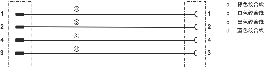
接线图
