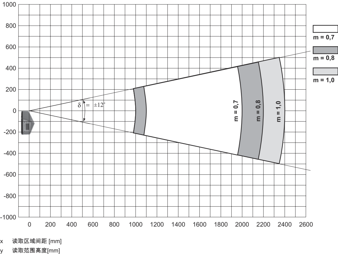
侧面条码阅读曲线
