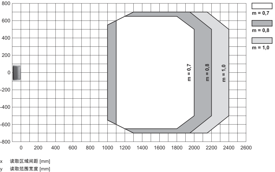
读取区域曲线
