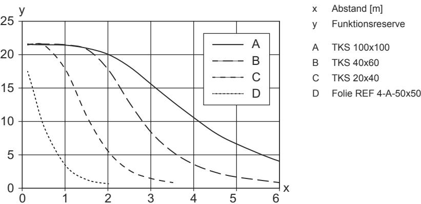
Typ. Funktionsreserve
