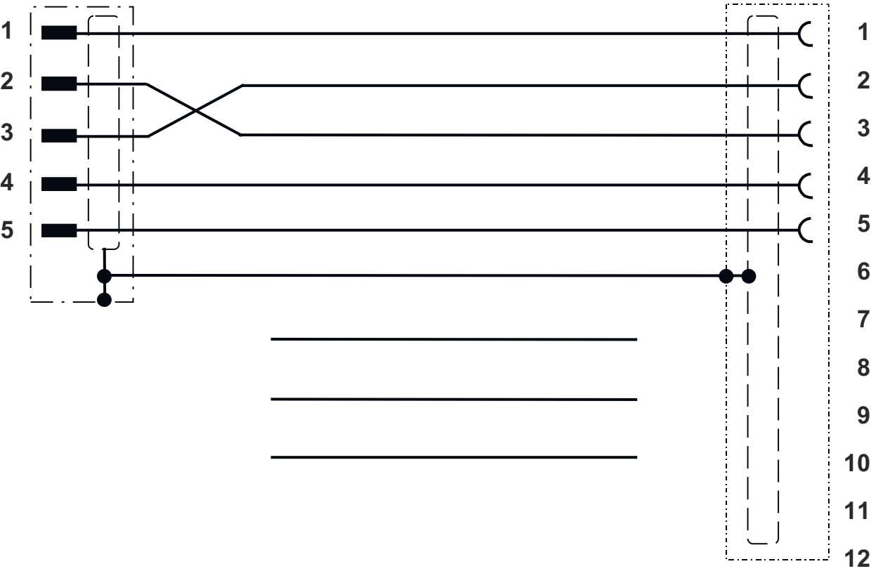
Esquema de fiação
