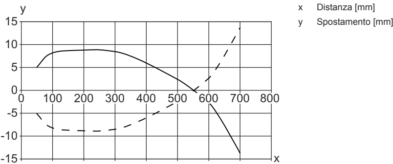
Comport. di risposta tip. (bianco 90%)
