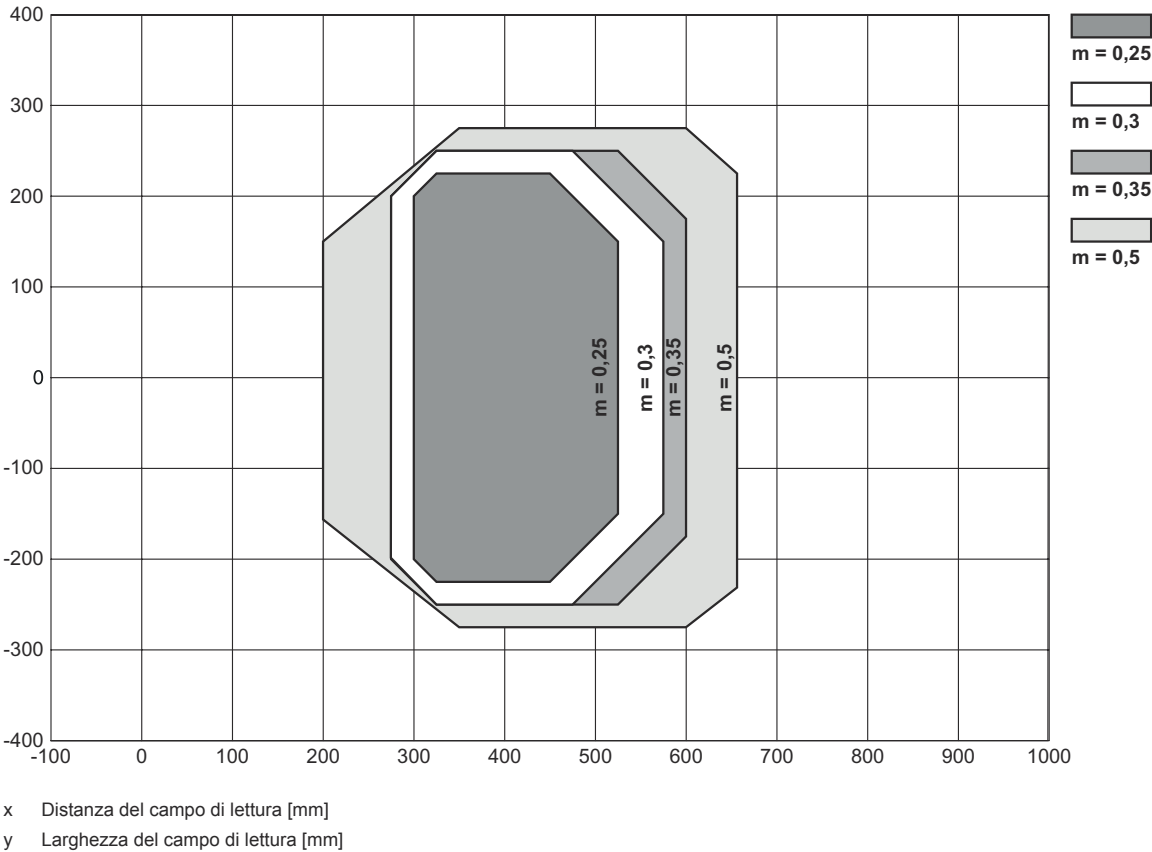
Curva del campo di lettura
