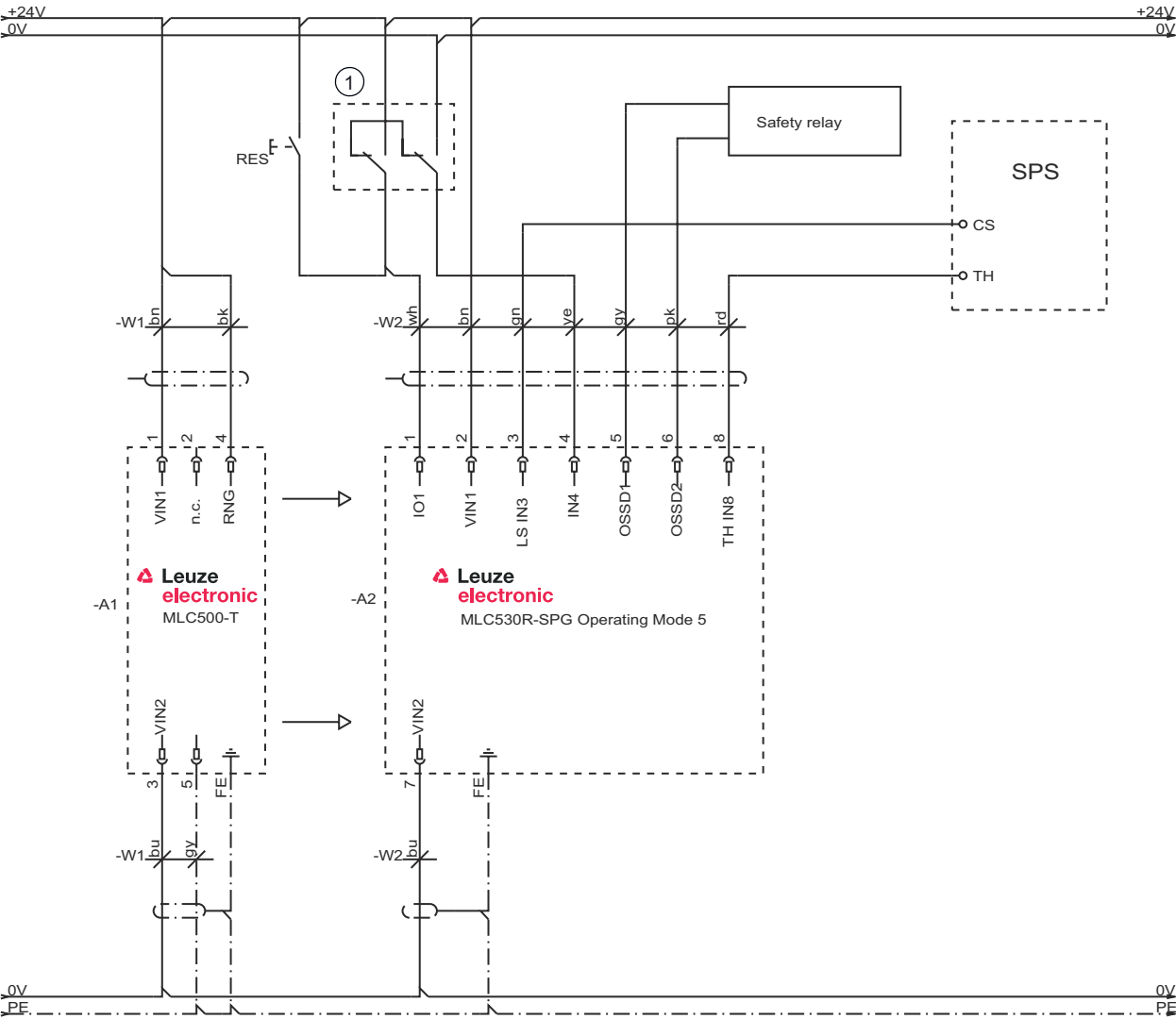
运行模式 5：含智能过程门控 (SPG) 的接线示例
