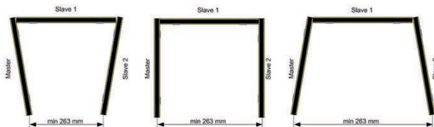
Bild 8.3: Mindestabstand für das Cascade-System
