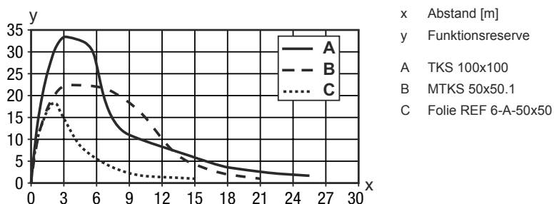
Typ. Funktionsreserve
