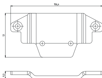
Fig. 14.2: Sistema de montagem BTU 500M
