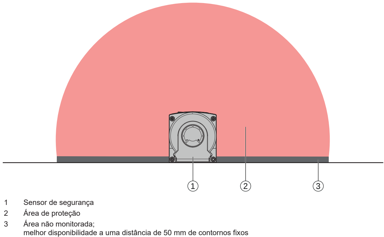
Fig. 6.4: Área não monitorada
