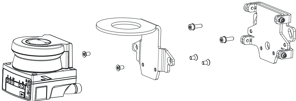
Fig. 6.16: Montagem com suporte de parede e estribo de proteção
