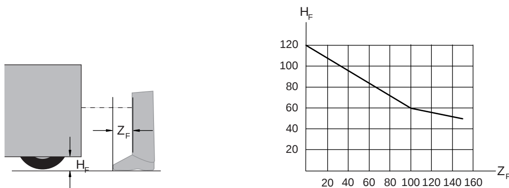
Fig. 6.13: Diagrama de determinação do suplemento Z_F na falta de distância ao chão H_F
