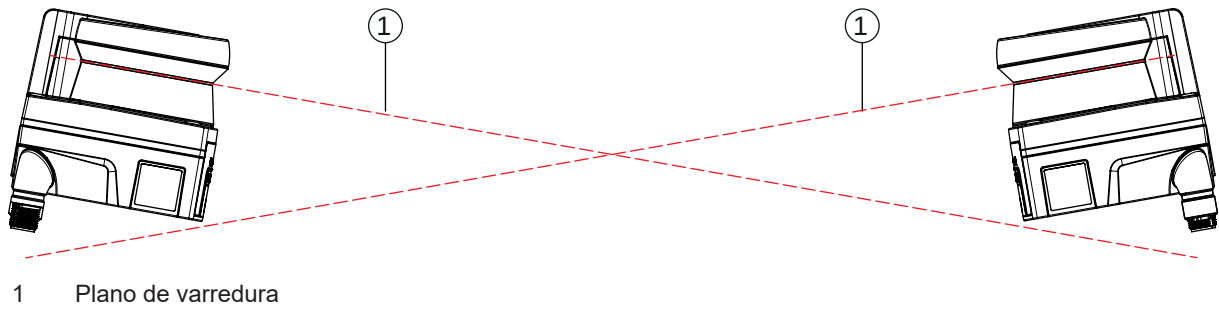
Fig. 6.9: Montagem em posições opostas, sem desfasamento vertical, alinhamento cruzado
