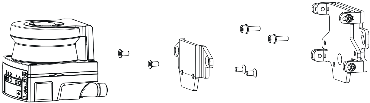
Fig. 6.15: Montagem com suporte de parede
