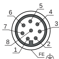
Fig. 7.2: Pinagem Conector M12, de 8 polos
