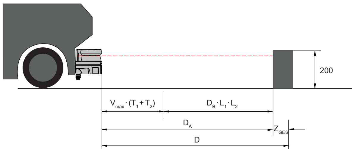
Fig. 6.12: Proteção móvel de acesso a zonas de perigo, cálculo da distância mínima necessária D
