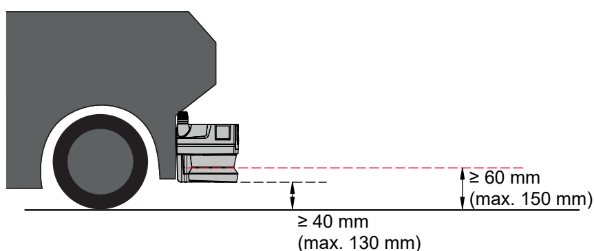
Fig. 6.11: Altura de montagem recomendada para RSL 210, RSL 220 e RSL 230 para sistemas de transporte não tripulados (utilização da função de segurança)
