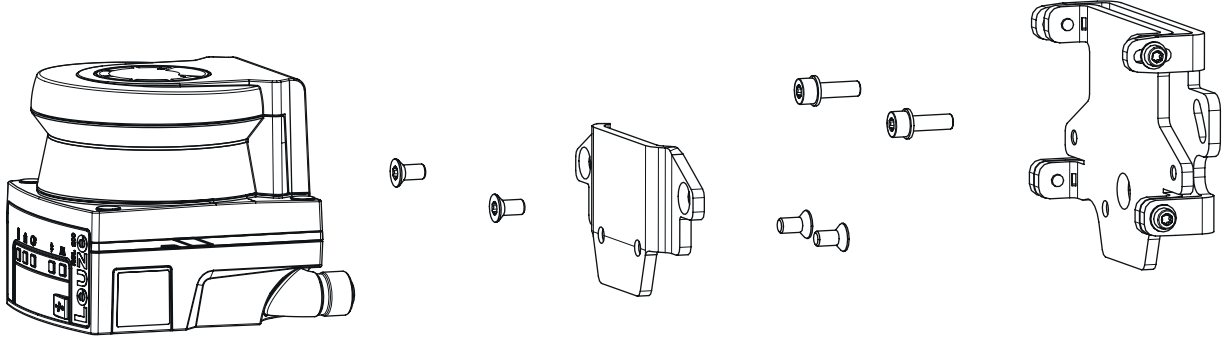
Resim 6.16: Duvar braketini sistem tarafına monte edin
