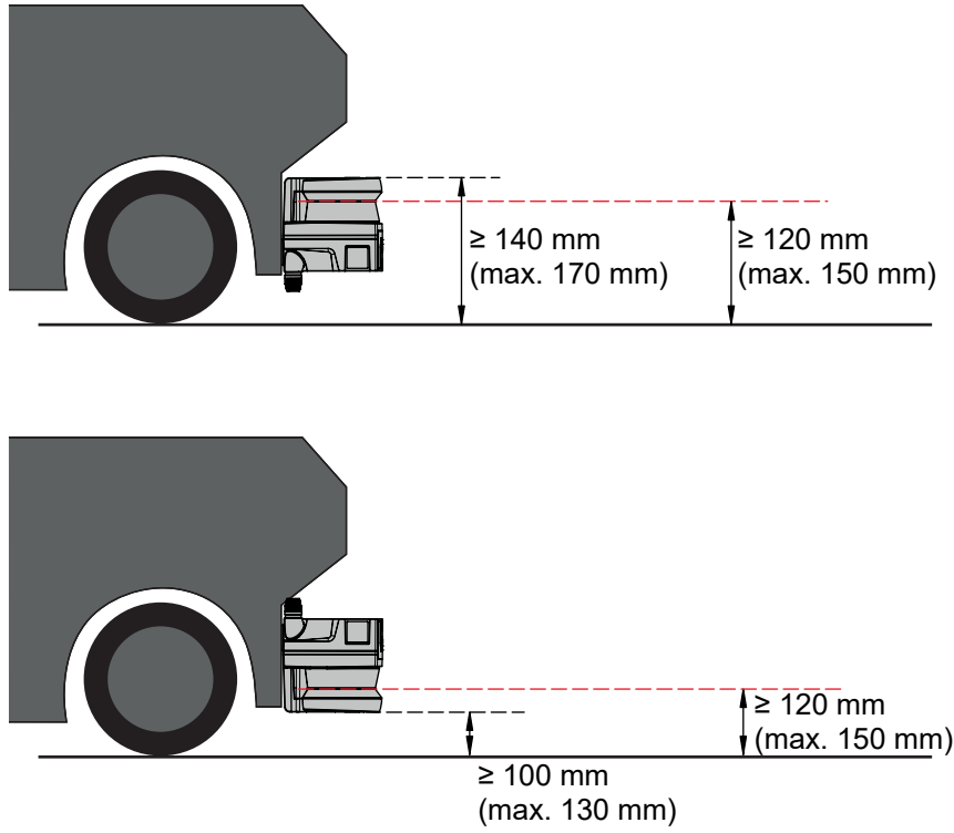
Resim 6.12: Sürücüsüz taşıma sistemleri için RSL 235 için önerilen montaj yüksekliği (navigasyon desteği için güvenlik işlevinin ve ölçüm veri çıkışının kullanımı)
