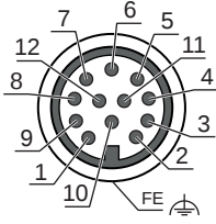
Resim 7.2: M12 konnektör, 12 kutuplu, A kodlu bağlantı yerleşimi
