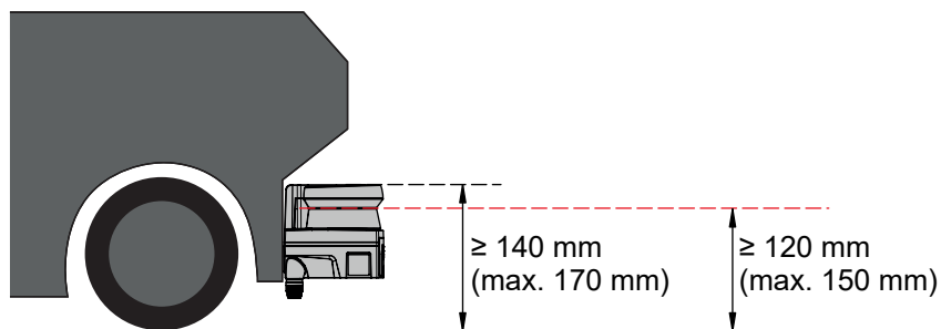
Fig. 6.11: Altura de montagem recomendada para RSL 210, RSL 220 e RSL 230 para sistemas de transporte não tripulados (utilização da função de segurança)
