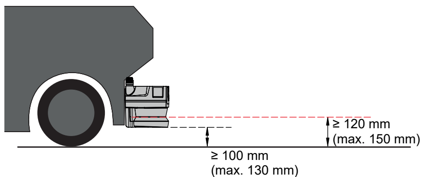
Fig. 6.12: Altura de montagem recomendada para o RSL 235 para sistemas de transporte não tripulados (utilização da função de segurança e saída de dados de medição para suporte à navegação)
