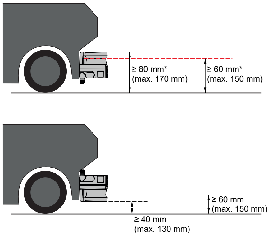
Fig. 6.11: Hauteur de montage recommandée pour RSL 210, RSL 220 et RSL 230 pour les systèmes de transport sans conducteur (utilisation de la fonction de sécurité)
