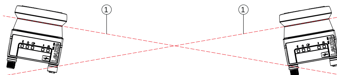
Fig. 6.8: Montage côte à côte, sans décalage en hauteur, alignement croisé
