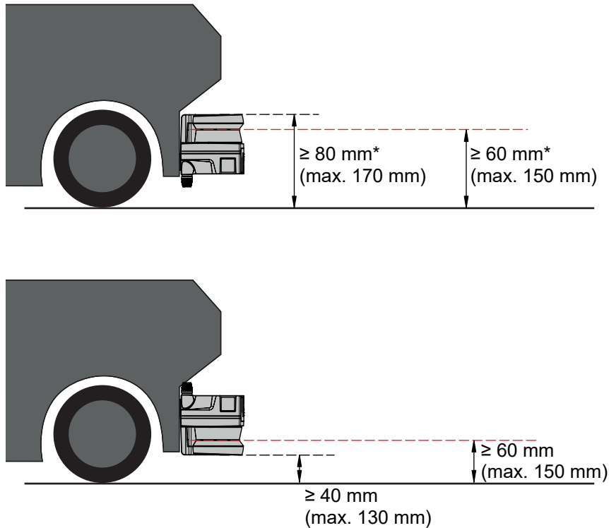
Figura 6.11: Altura de montaje recomendada para RSL 210, RSL 220 y RSL 230 en sistemas de transporte sin conductor (uso de la función de seguridad)
