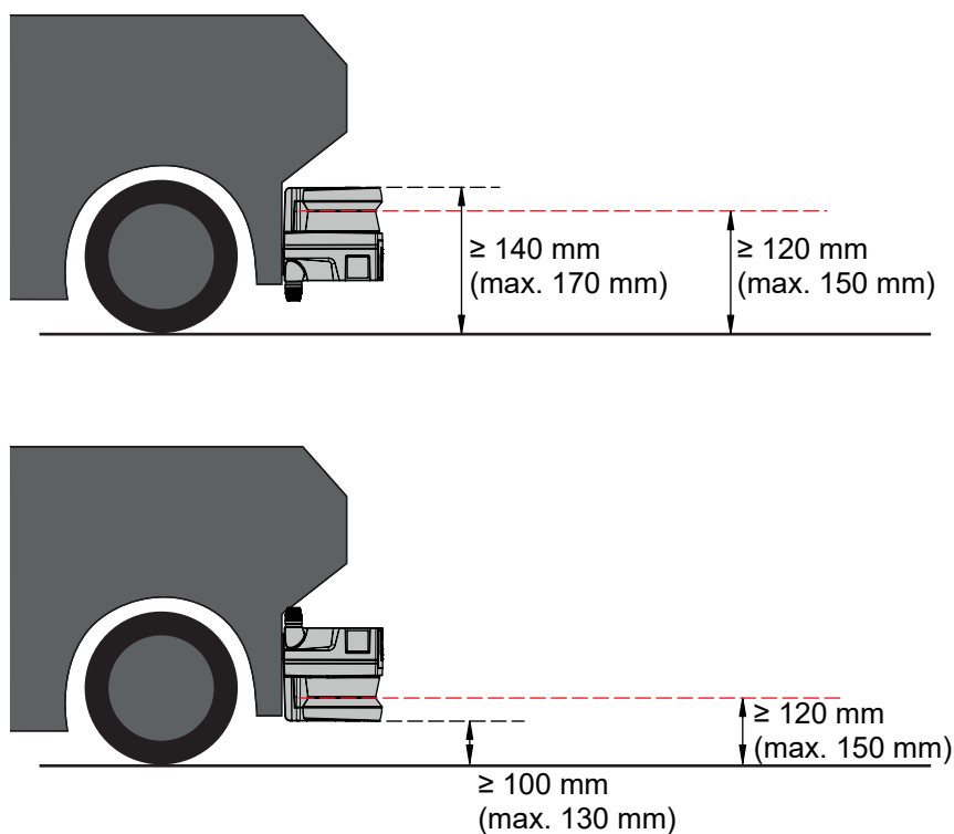
Figura 6.12: Altura de montaje recomendada para RSL 235 en sistemas de transporte sin conductores (uso de la función de seguridad y de la salida de datos de medición para la asistencia para la navegación)
