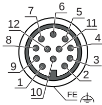
Bild 7.2: Anschlussbelegung M12-Stecker, 12-polig
