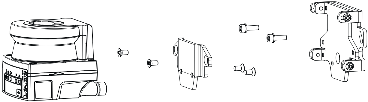
Fig. 6.15: Montage avec support mural
