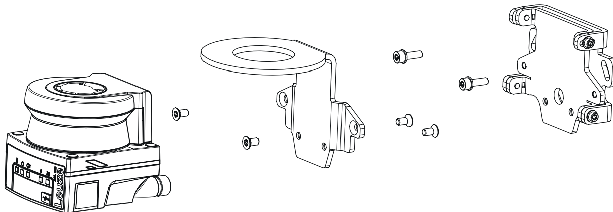
Fig. 6.16: Montage avec support mural et support de protection
