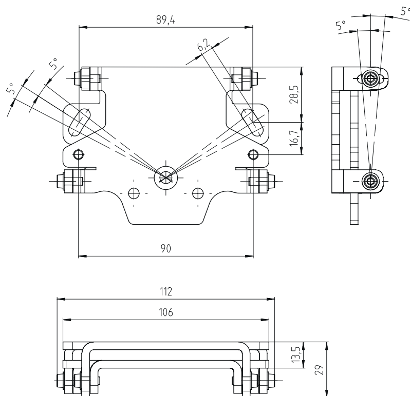
Fig. 14.2: Système de montage BTU 500M
