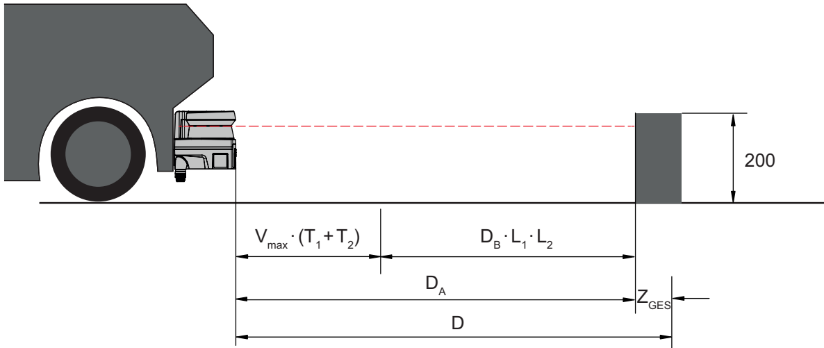
Bild 6.12: Mobile Gefahrenbereichssicherung, Berechnung der erforderlichen Mindestdistanz D
