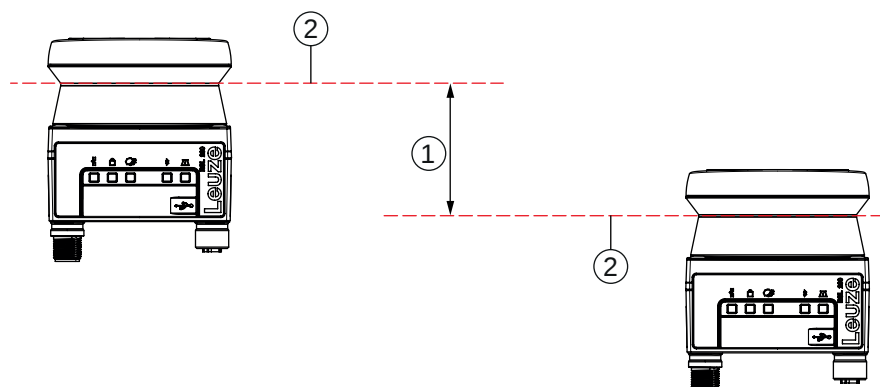
Bild 6.6: Abschirmung gegen Beeinflussung benachbarter Schutzfelder
