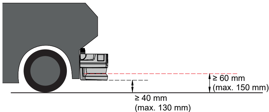
Bild 6.11: Empfohlene Montagehöhe für RSL 210, RSL 220 und RSL 230 bei fahrerlosen Transportsystemen (Nutzung der Sicherheitsfunktion)
