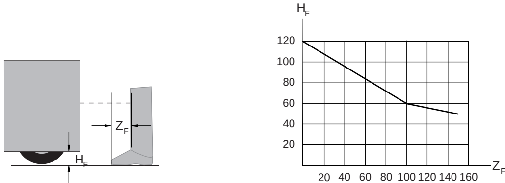
Resim 6.13: İlave yük Z_F 'nin kötü zemin serbestliği H_F 'de belirlenmesi için diyagram
