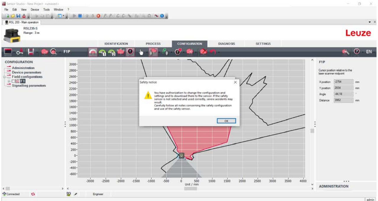
Resim 8.37: Güvenlik konfigürasyonunu indirmeden önce kontrol
