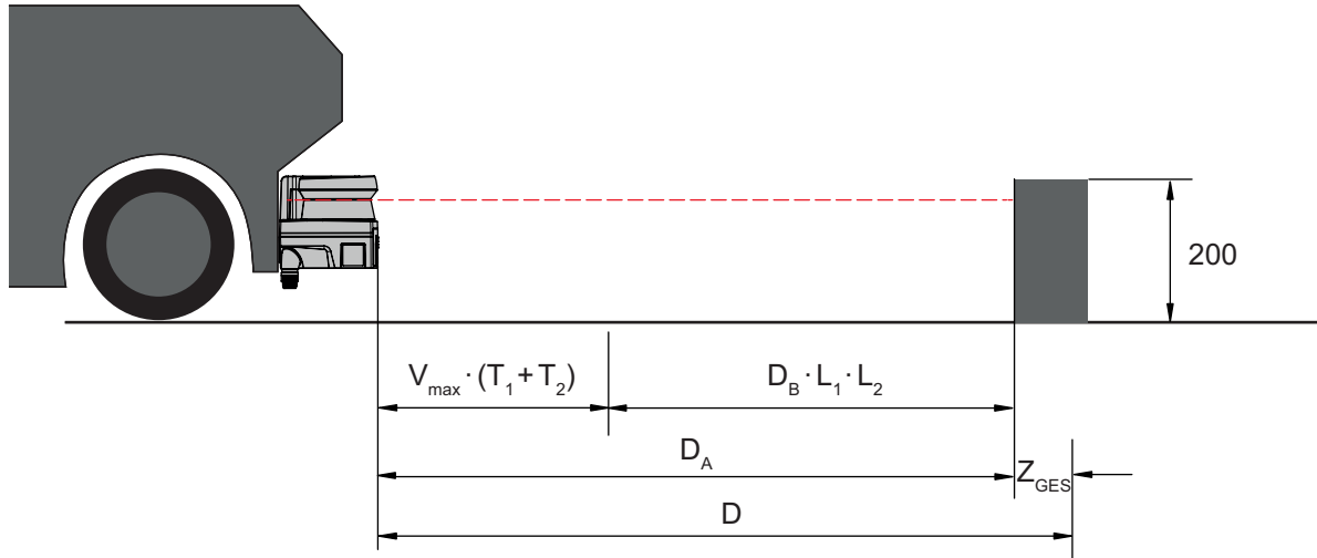
Resim 6.12: Mobil tehlike alanı emniyeti, gerekli asgari mesafe D'nin hesaplanması
