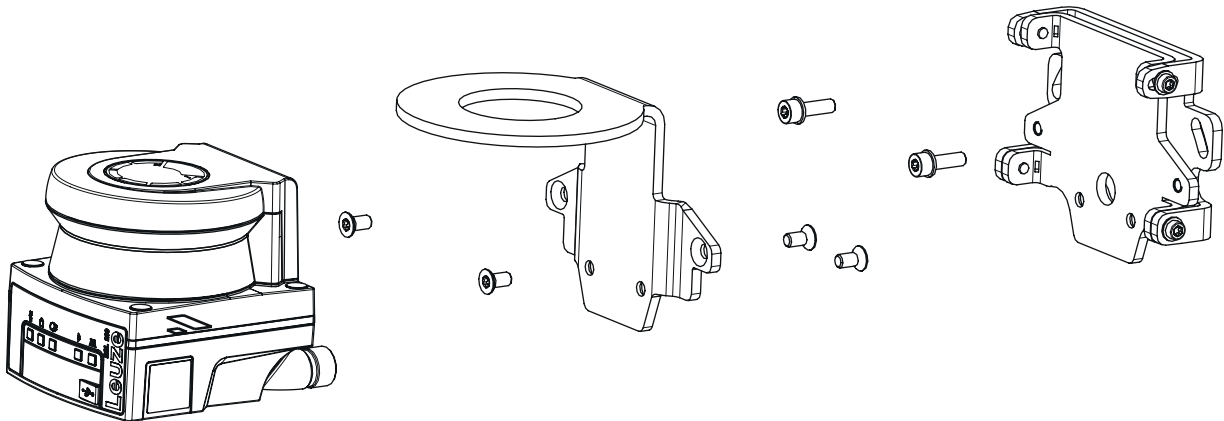
Resim 6.16: Duvar braketini ve koruyucu braket ile montaj
