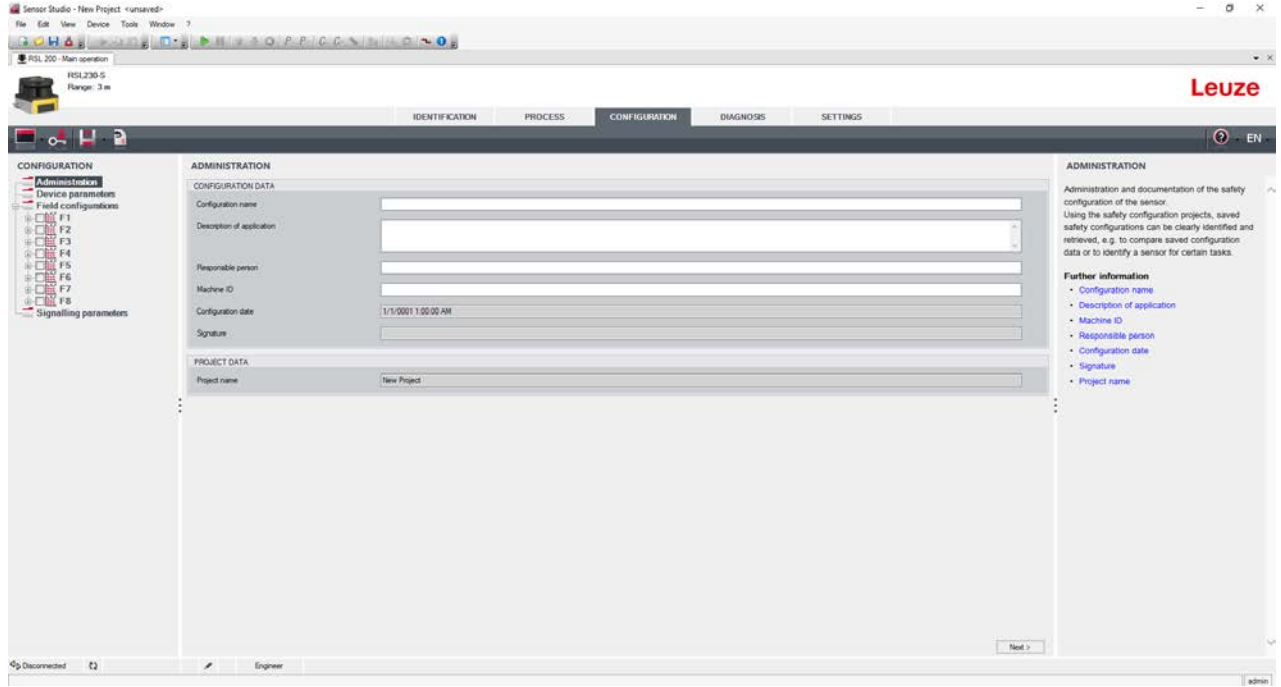
Resim 8.34: Konfigürasyon projesi için başlangıç ekranı
