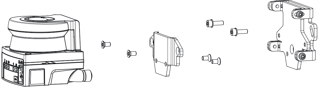
Resim 6.15: Duvar braketini sistem tarafına monte edin
