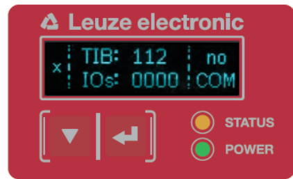
Figure 3.6 : Touches de fonction sur le récepteur
