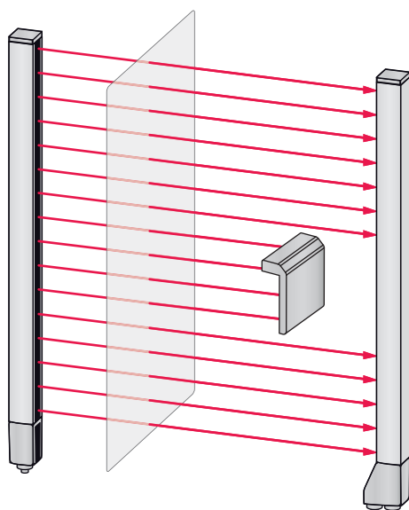
Figure 11.3 : Rayonnement sûr à travers des films laiteux
