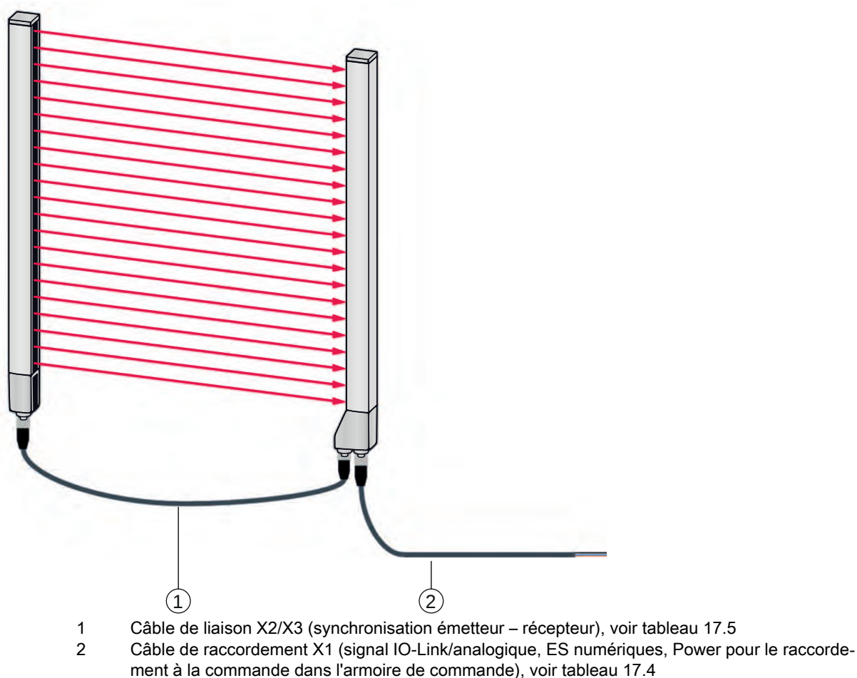
Figure 17.2 : Interface IO-Link (analogique)
