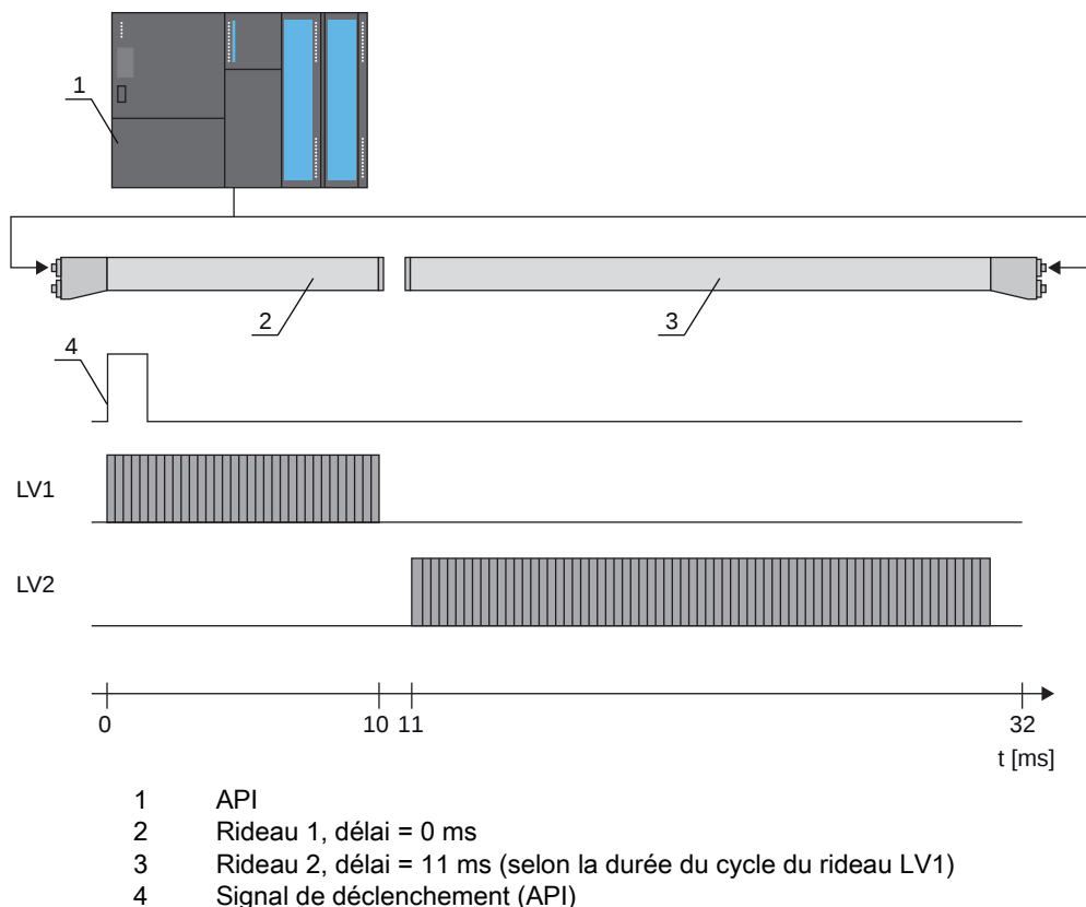
Figure 4.12 : Commande par déclenchement externe
