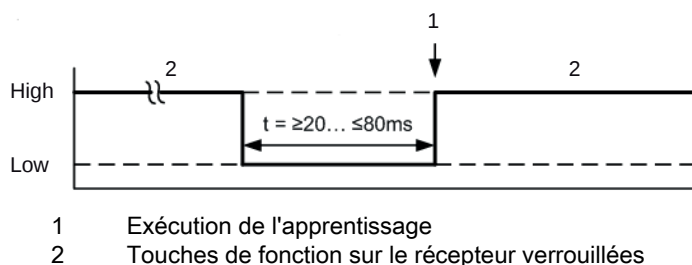
Figure 8.5 : Signaux de commande en cas d'apprentissage par bouton déporté avec configuration PNP
