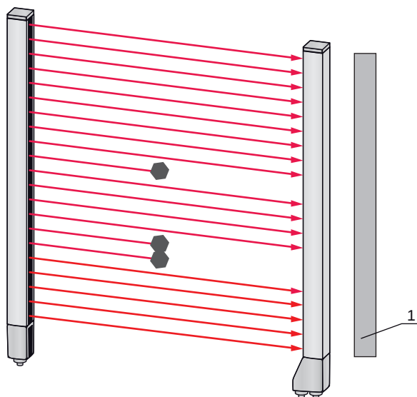
Figure 4.8 : Configuration de lissage "3", mais seulement deux faisceaux voisins sont interrompus au maximum
