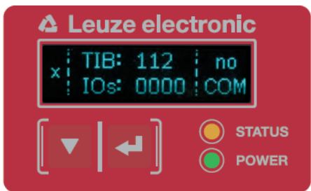
Figure 8.3 : Représentation à l'écran de l'état du mode de processus du rideau lumineux
