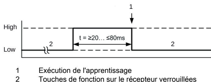
Figure 8.6 : Signaux de commande en cas d'apprentissage par bouton déporté avec configuration NPN
