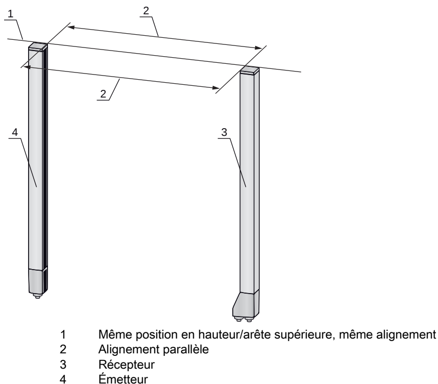
Figure 6.1 : Disposition de l'émetteur et du récepteur
