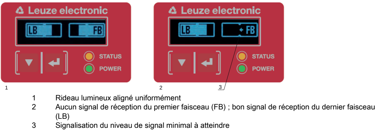
Figure 3.4 : Écran OLED sur le récepteur en mode d'alignement
