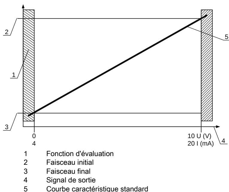
Figure 9.1 : Courbe caractéristique de la sortie analogique (courbe caractéristique standard)
