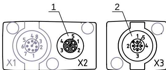
Figure 7.7 : Connexion X2/X3– CML 700i avec interface IO-Link/analogique
