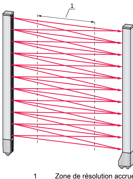
Figure 4.3 : Parcours du faisceau en type de balayage "Croisé"
