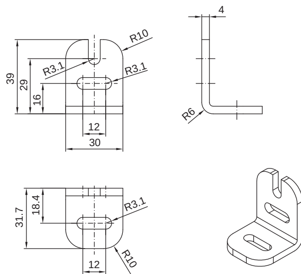
Figura 20.3: Supporto angolare BT-2L
