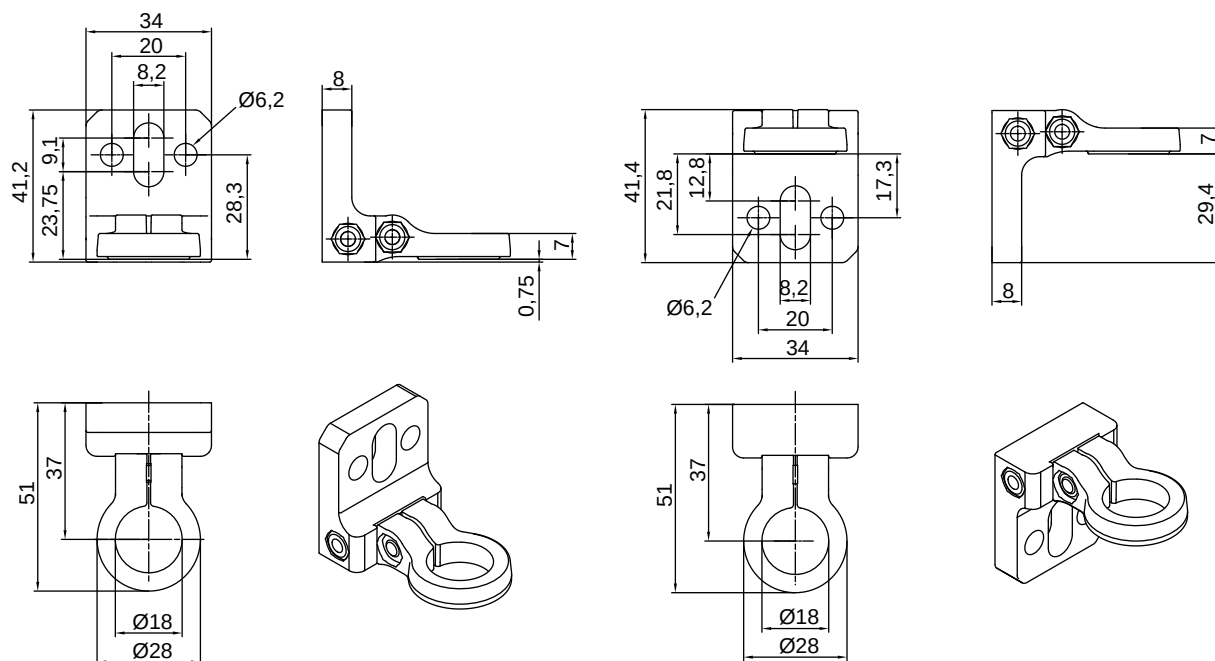
Figura 20.5: Supporto girevole BT-2R1 (in due viste di montaggio)
