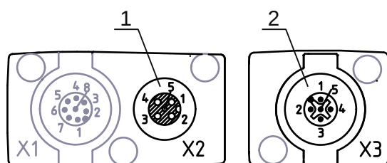
Figura 7.8: Collegamento X2/X3- CML 700i con interfaccia IO-Link/analogica
