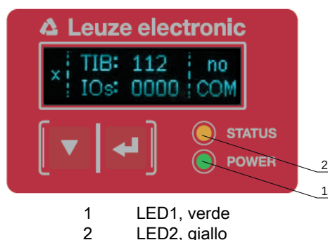
Figura 3.3: Indicatori a LED sul ricevitore
