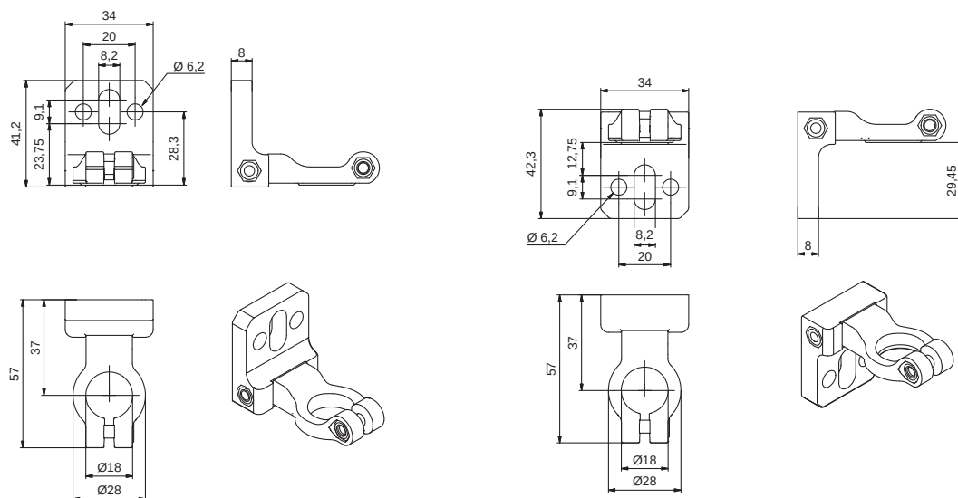
Figura 20.6: Supporto girevole BT-2HF
