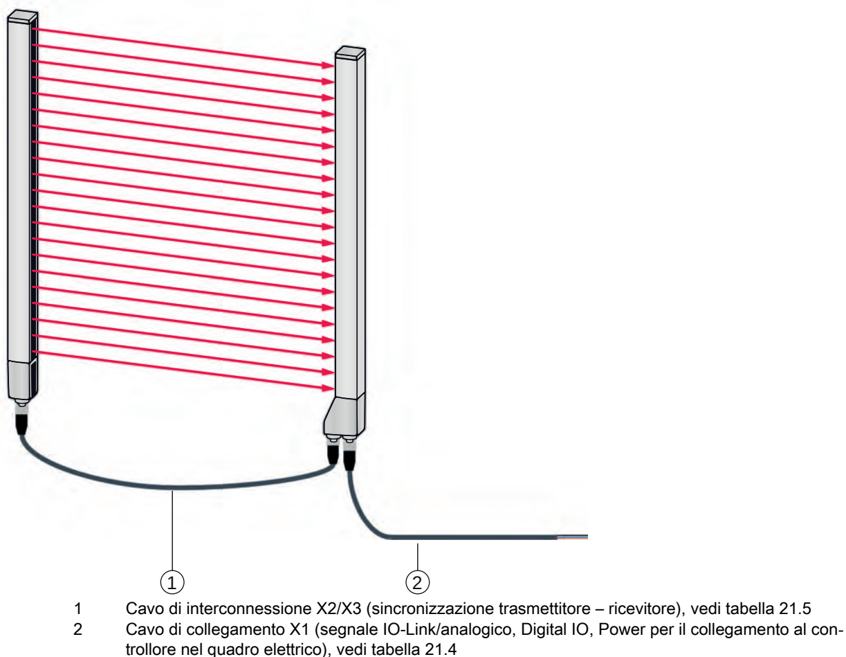
Figura 21.2: Interfaccia IO-Link (analogica)
