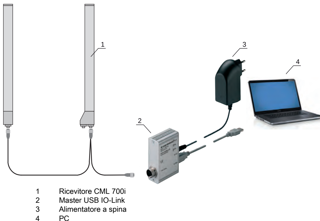
Figura 16.3: Collegamento della CML 700i (fieldbus) al master USB IO-Link
