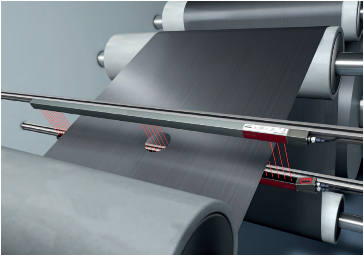
Figura 5.6: Riconoscimento fori
