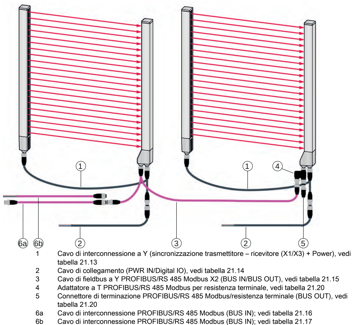
Figura 21.6: Interfaccia PROFIBUS o RS 485 Modbus (resistenza terminale alternativa)
