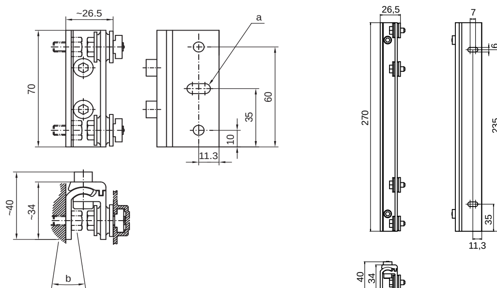
Figura 20.7: Supporti orientabili BT-2SSD e BT-2SSD-270
