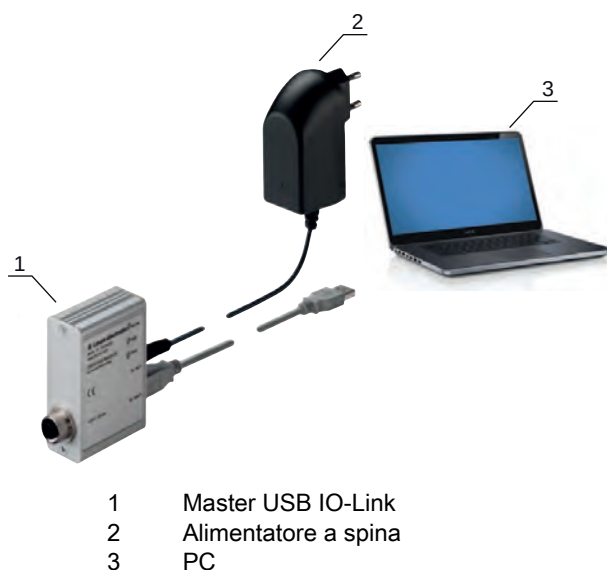
Figura 16.1: Collegamento al PC via master USB IO-Link
