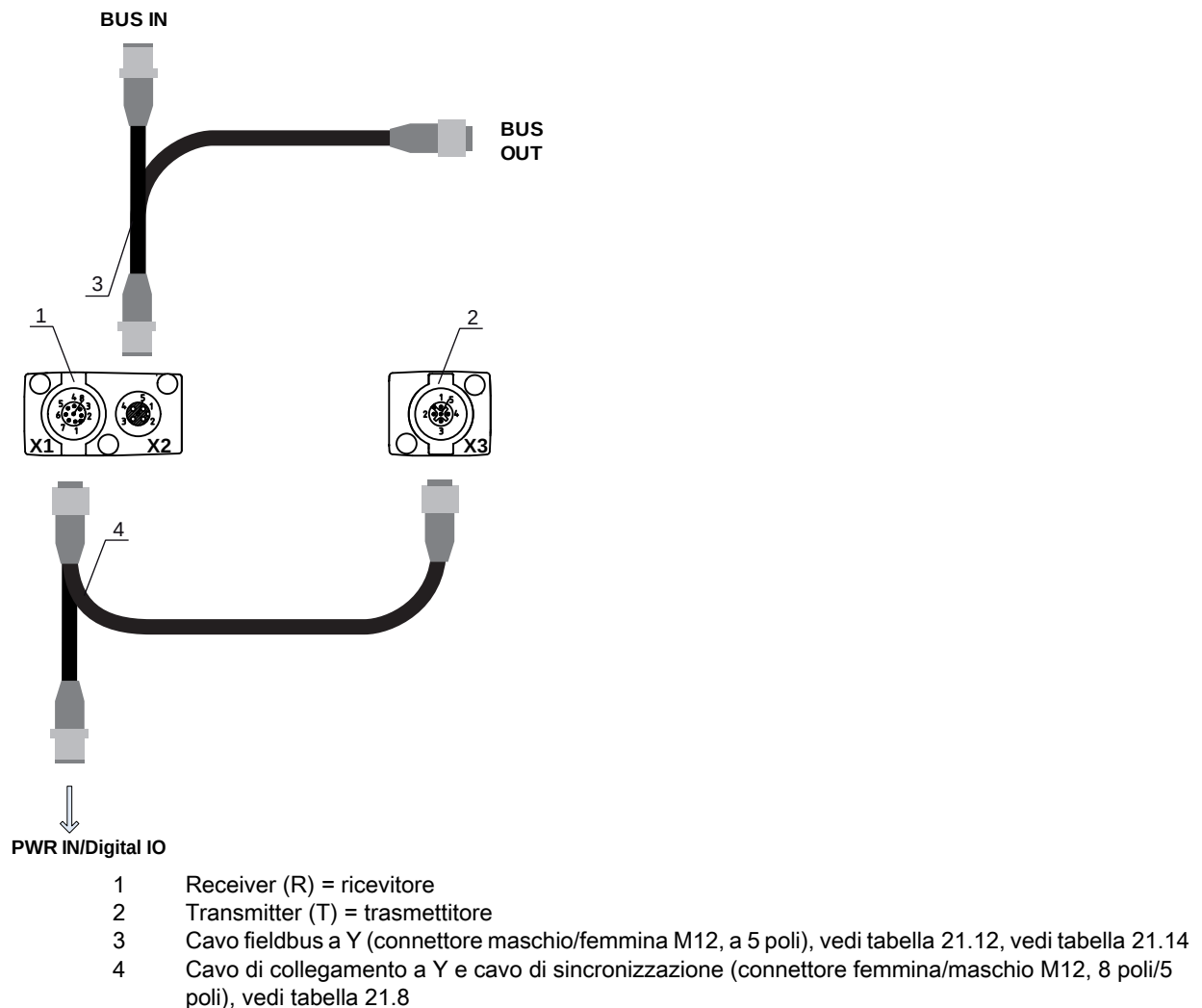
Figura 7.9: Collegamento elettrico – CML 700i con interfaccia CANopen, PROFIBUS e RS 485 Modbus
