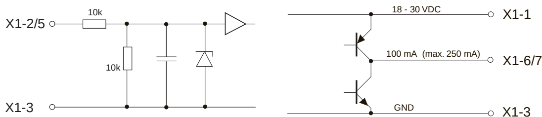
Figura 7.4: Rappresentazione del principio di ingressi/uscite digitali
