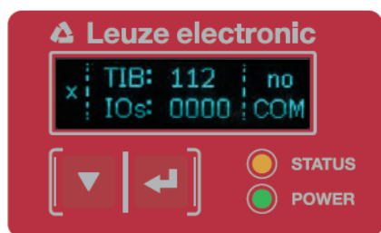
Figura 3.7: Tasti funzione sul ricevitore
