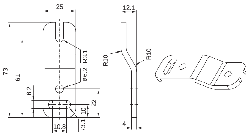
Figura 20.4: Supporto parallelo BT-2Z
