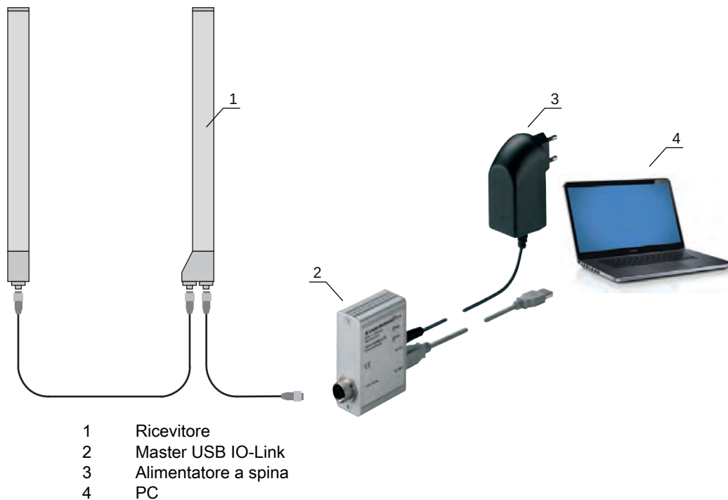
Figura 16.2: Collegamento della CML 700i (analogico/IO-Link) al master USB IO-Link
