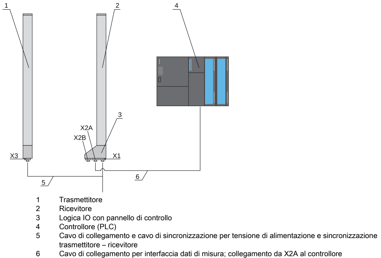
Figura 3.2: Sistema PROFINET in interazione con un PLC
