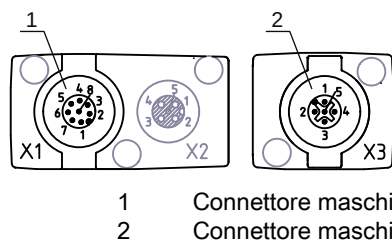
Figura 7.10: Collegamento X1/X3 – CML 700i con interfaccia CANopen, PROFIBUS e RS 485 Modbus
