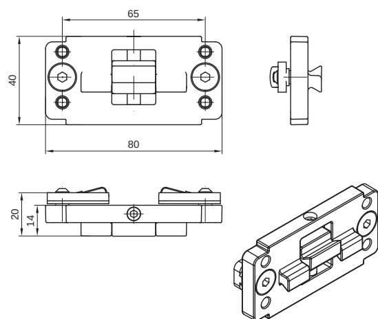
Figura 20.9: Supporto di serraggio BT-2P40
