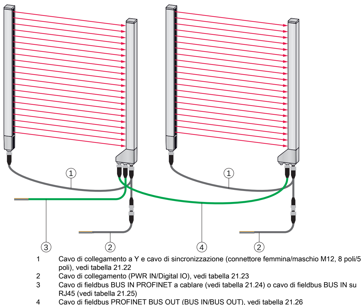
Figura 21.7: Interfaccia PROFINET
