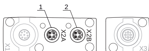
Figura 7.17: Collegamenti X2 – CML 700i con interfaccia PROFINET
