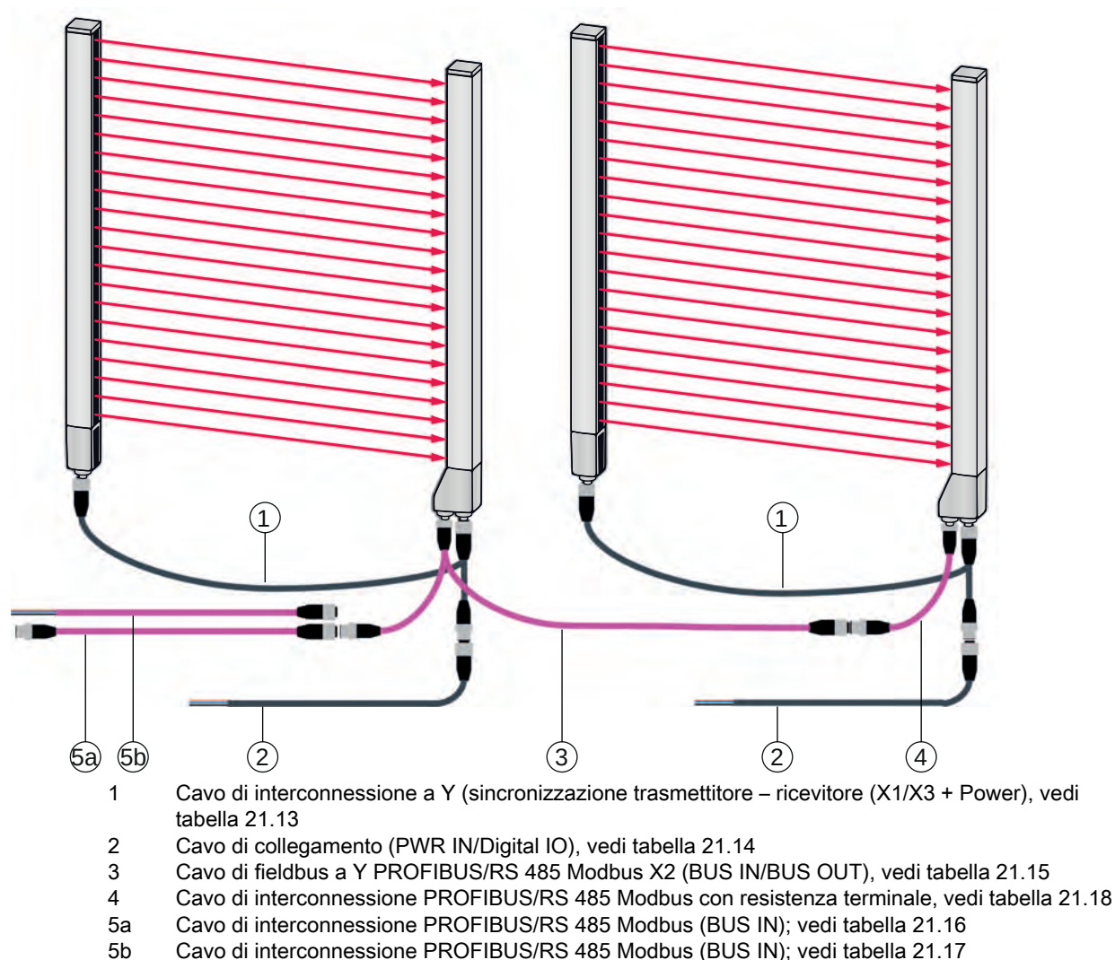
Figura 21.5: Interfaccia PROFIBUS o RS 485 Modbus
