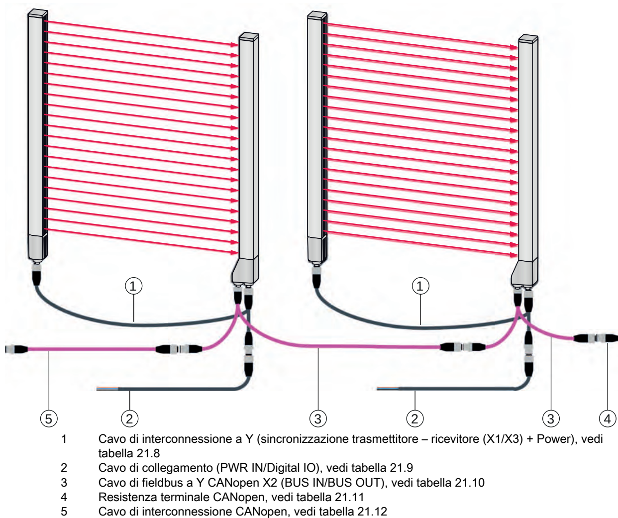
Figura 21.4: Interfaccia CANopen
