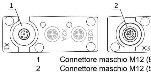
Figura 7.15: Collegamento X1/X3 – CML 700i con interfaccia PROFINET
