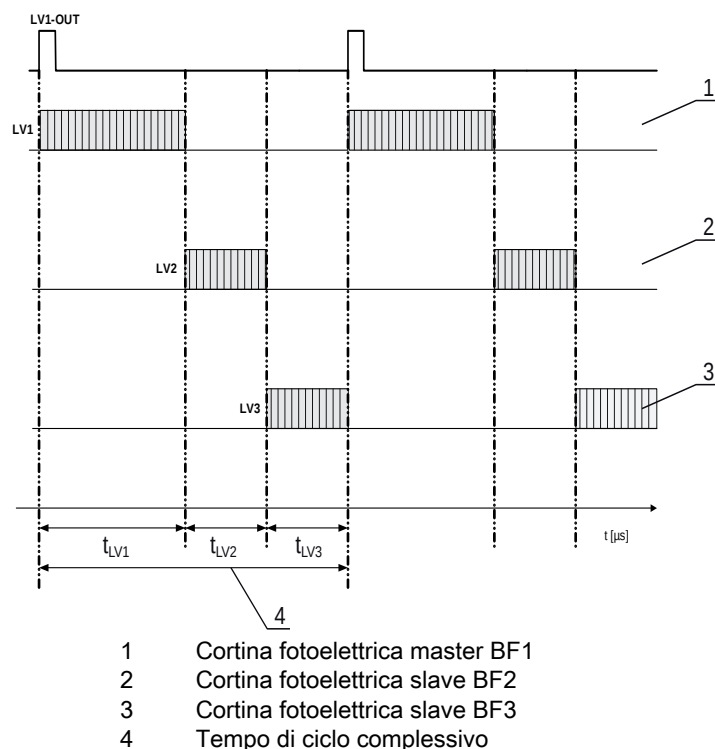
Figura 15.1: Esempio: collegamento in cascata con tre cortine fotoelettriche
