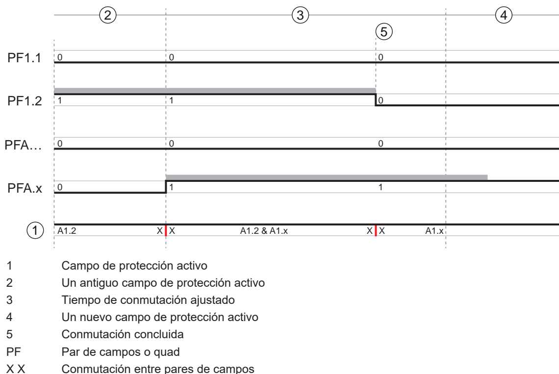
Figura 5.3: Diagrama de tiempos y señales: supervisión solapada
