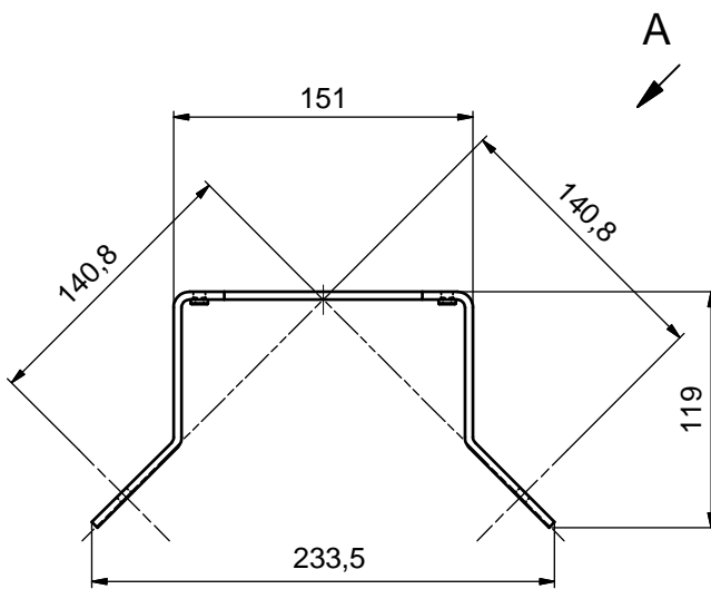
Figura 15.11: Escuadra de montaje BT840M, vista A
