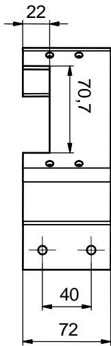
Figura 15.11: Escuadra de montaje BT840M, vista A
