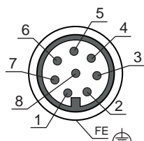
Figura 8.1: Assegnazione dei pin del sensore di sicurezza
