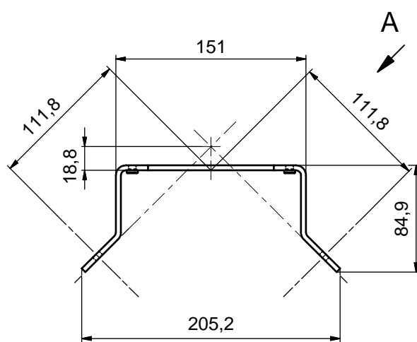
Figura 15.8: Staffa di protezione BTP800M
