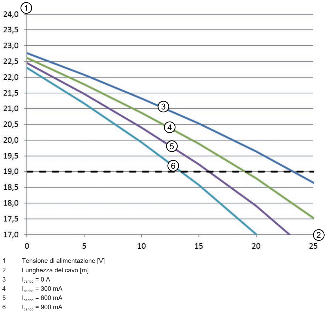
Figura 8.4: Diagramma per la stima delle cadute di tensione sulla linea di alimentazione
