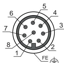
Fig. 8.1: Affectation des raccordements du capteur de sécurité
