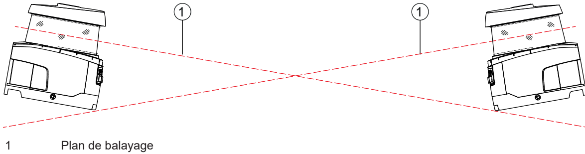
Fig. 7.11: Montage opposé, sans décalage en hauteur, alignement croisé
