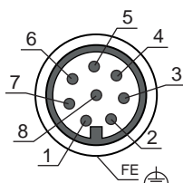
Figura 8.1: Asignación de pines del sensor de seguridad
