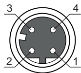
Figura 8.2: Asignación de pines de la interfaz Ethernet
