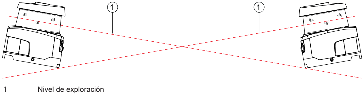
Figura 7.11: Montaje frontal, sin desfase de alturas, en orientación cruzada
