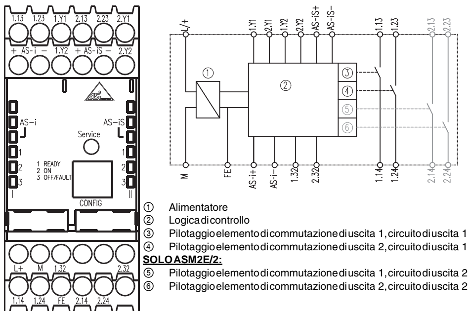
Figura 7.1: Disposizione dei morsetti / schema a blocchi monitor di sicurezza AS-interface ASM2E/1 e ASM2E/2
