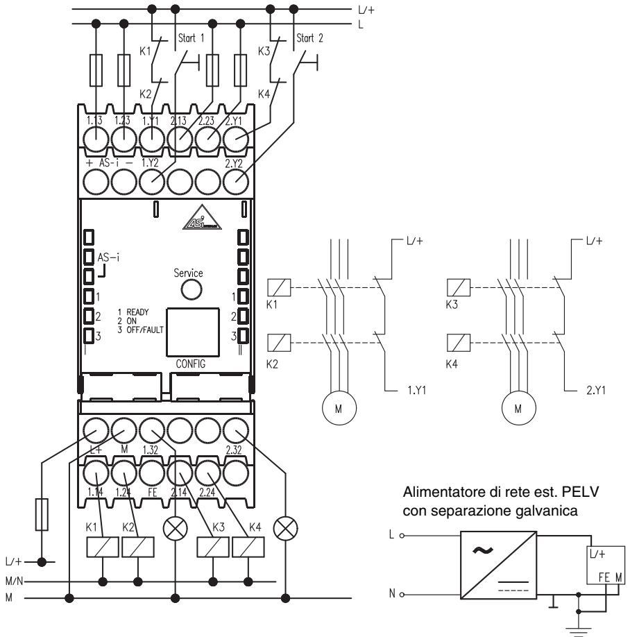
Figura 6.2: Schema dei collegamenti monitor di sicurezza AS-interface ASM1/2 e ASM1E/2
