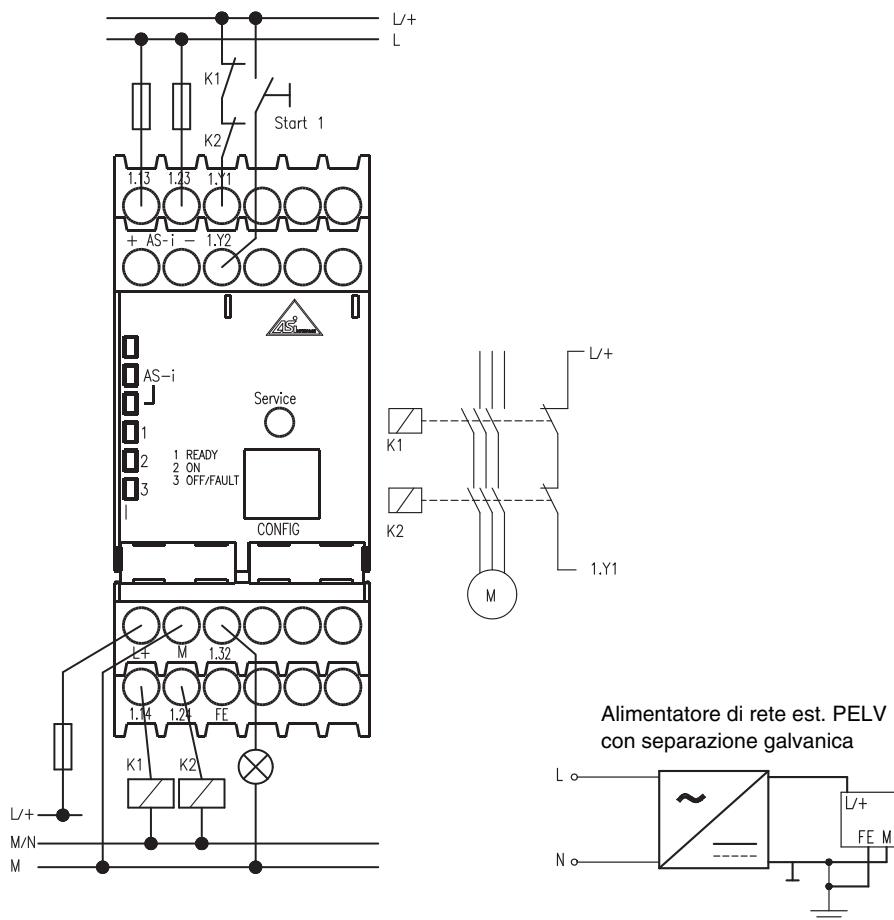
Figura 5.2: Schema dei collegamenti monitor di sicurezza AS-interface ASM1/1 e ASM1E/1
