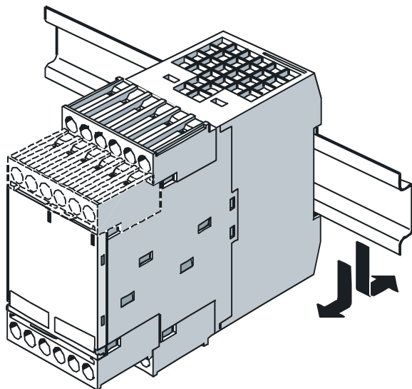
Figura 4.1: Montaggio
