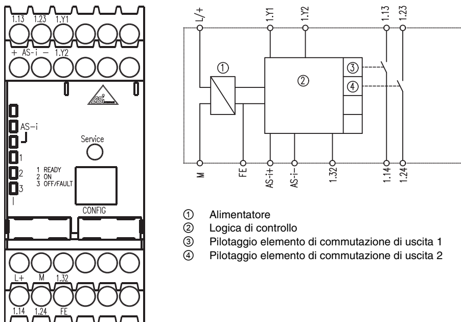
Figura 5.1: Disposizione dei morsetti / schema a blocchi monitor di sicurezza AS-interface ASM1/1 e ASM1E/1
