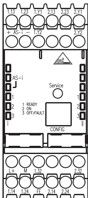
Figura 6.1: Disposizione dei morsetti / schema a blocchi monitor di sicurezza AS-interface ASM1/2 e ASM1E/2
