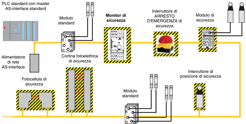
Figura 1.1: Componenti standard e riferiti alla sicurezza in una rete AS-interface
