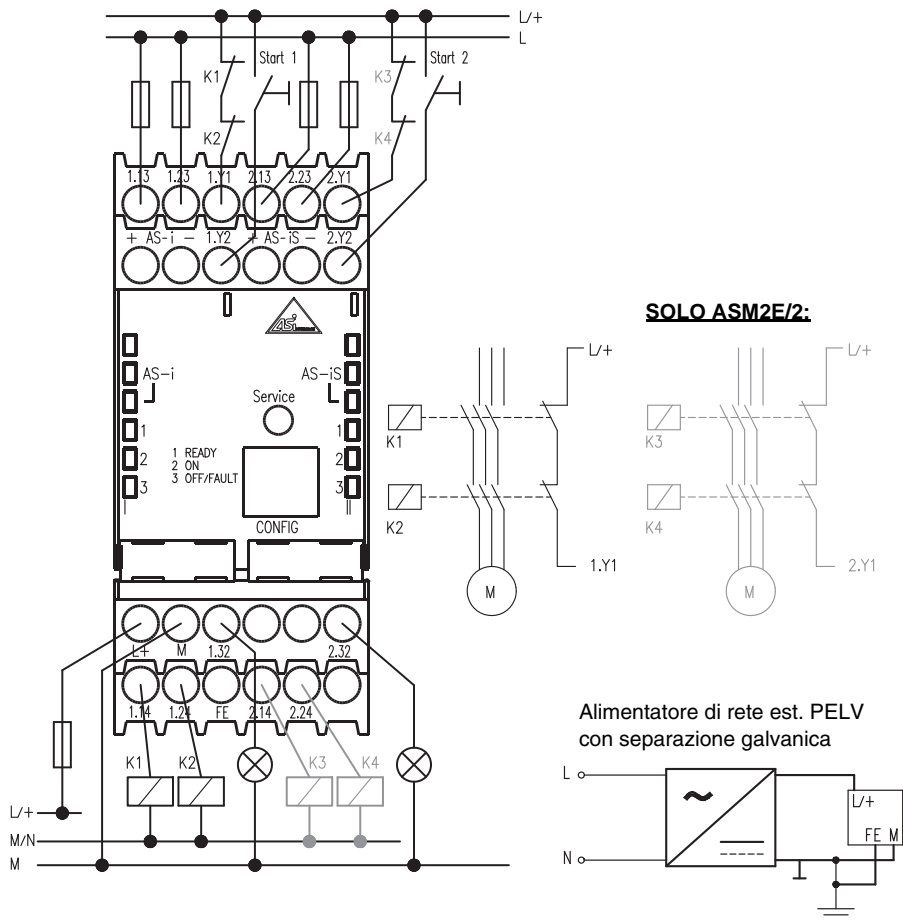
Figura 7.2: Schema dei collegamenti monitor di sicurezza AS-interface ASM2E/1 e ASM2E/2
