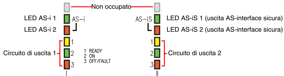
Figura 9.1: Tavola dei LED dell'apparecchio
