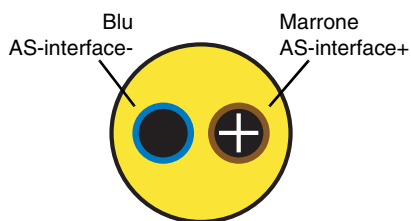
Cavo tondo AS-interface a due fili (consigliato: cavo flessibile per corrente forte H05VV-F2x1,5 secondo DIN VDE 0281)
