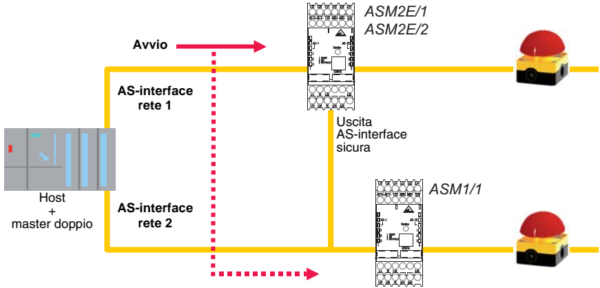
Figura 1.3: Esempio: sorveglianza di 2 gruppi di attuatori AS-interface decentralizzati
